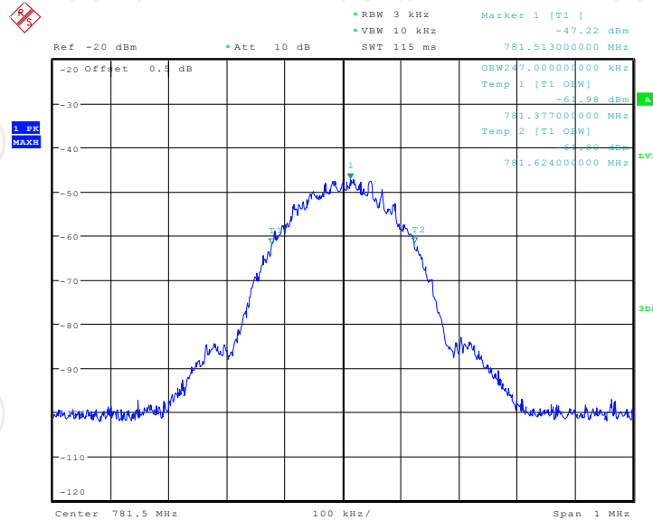
Band13 GSM UL Input
