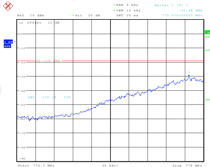
Band13 GSM UL Left Side Pre AGC+10dB
