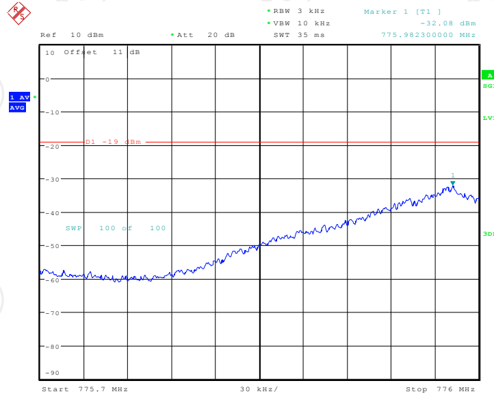
Band13 GSM UL Left Side Pre AGC
