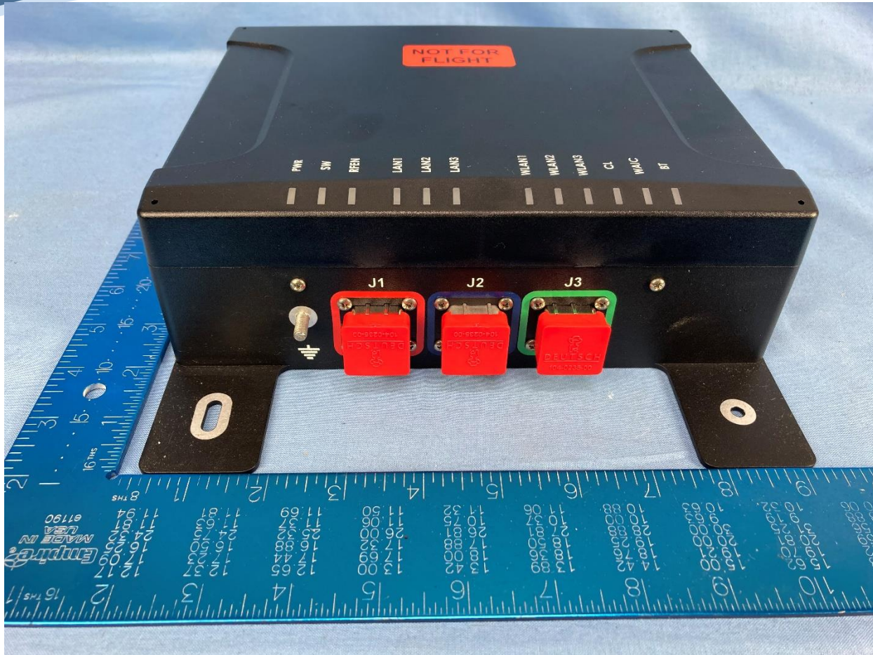
RaveAP_left
