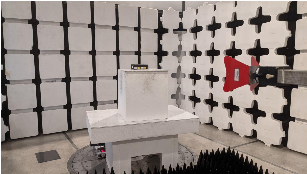
Emissions 1-18GHz
