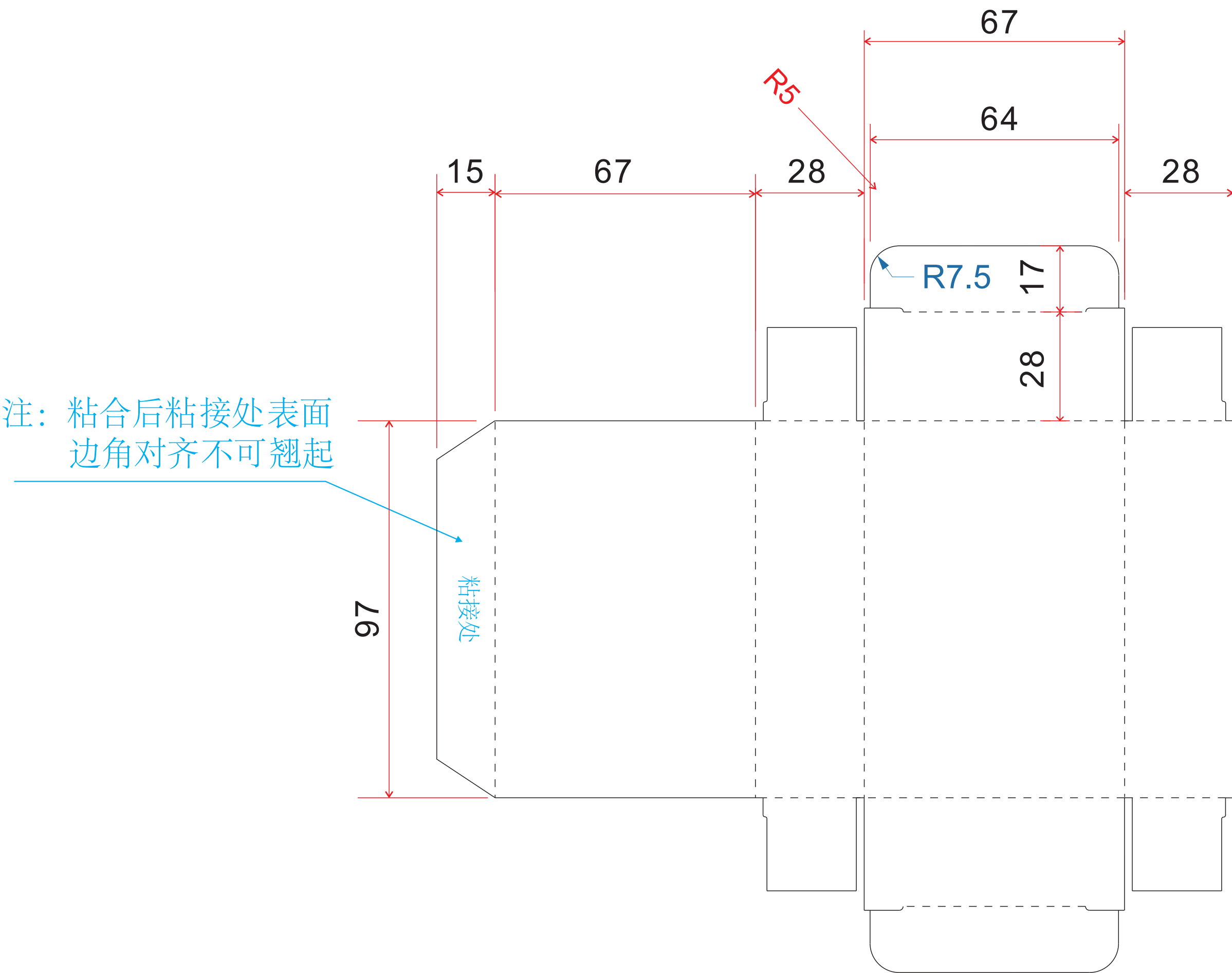
刀模图
