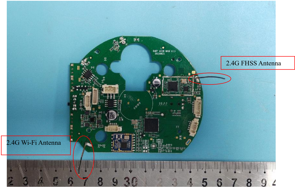
Antenna
