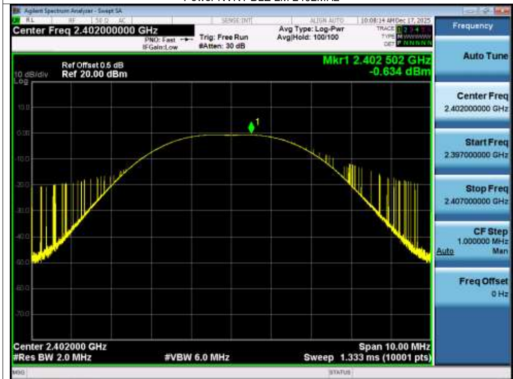
Power NVNT BLE 2M 2402MHz
