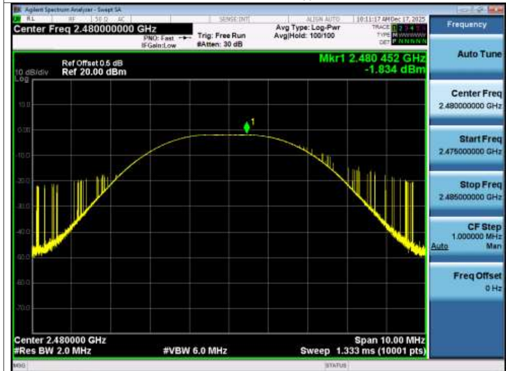
Power NVNT BLE 2M 2480MHz
