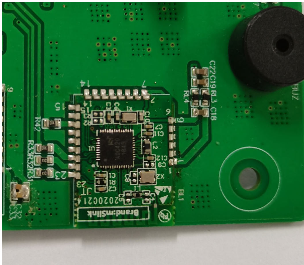
Bluetooth module
