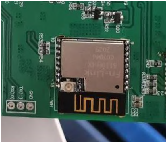
Wi-Fi module
