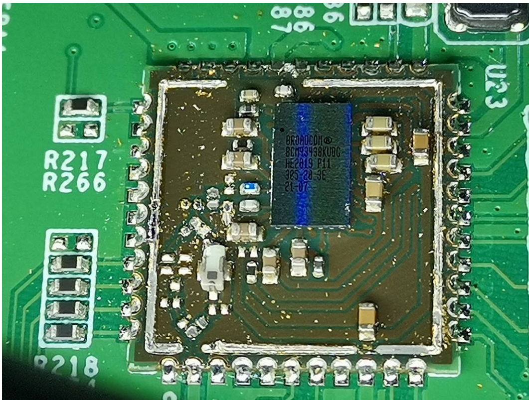
Wi-Fi Module
