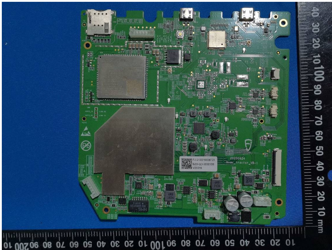
LTE Module
