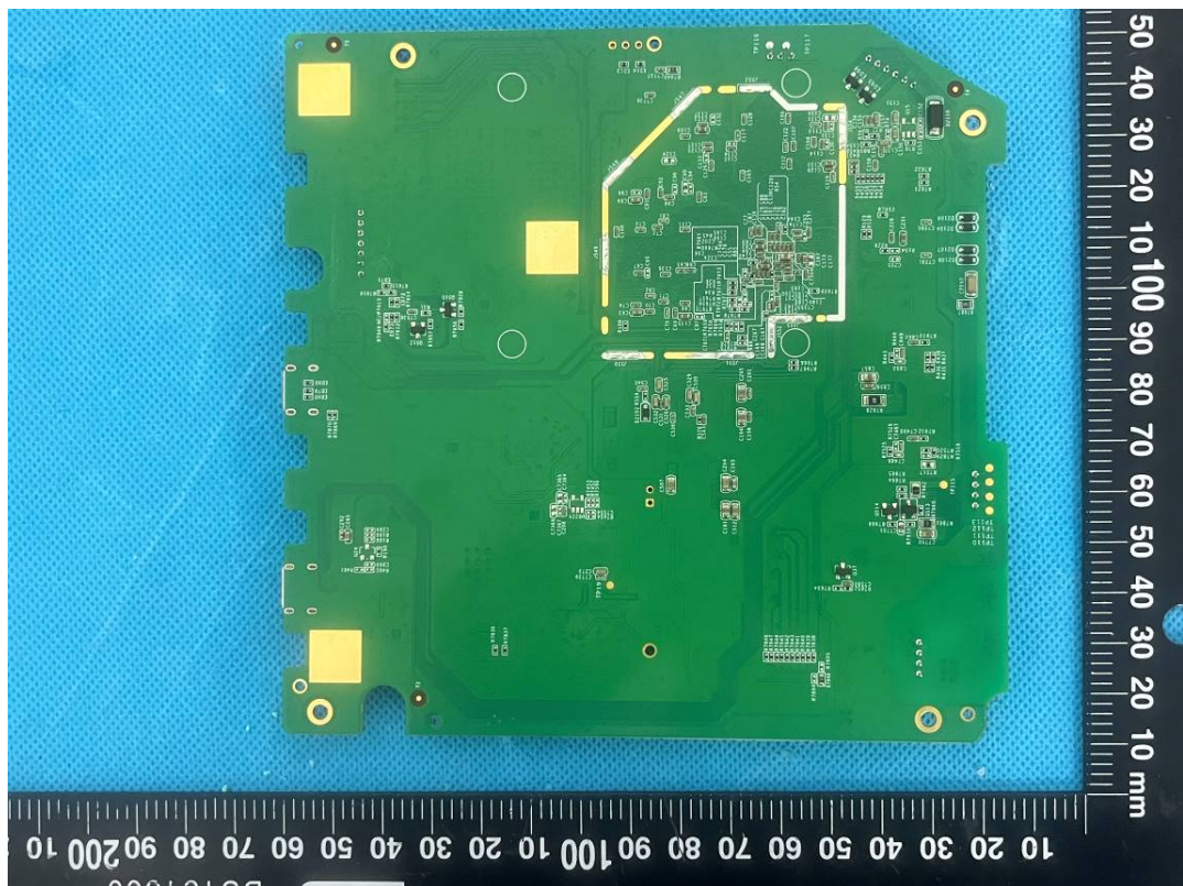
BT/WiFi Antenna
