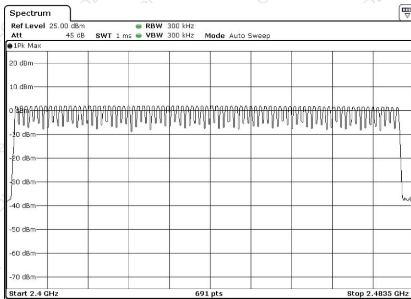
\pi/4 -DQPSK - 2-DH1 Test Plots
