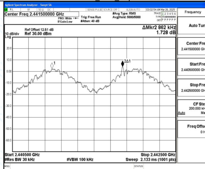
2DH5_Ant1_Hop
