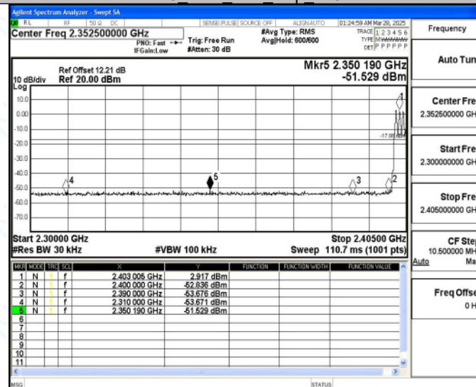
DH5_Ant1_Low_Hop_2402
