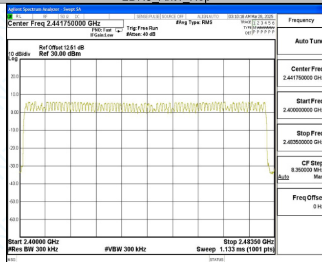
3DH5_Ant1_Hop
