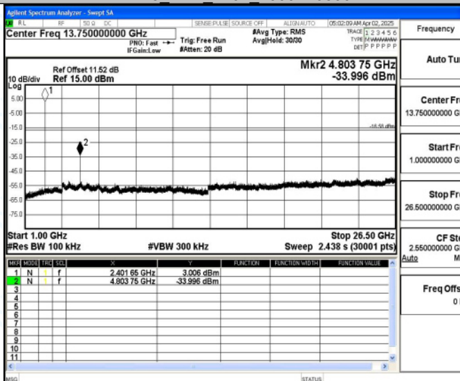
DH5_Ant1_2402_1000~26500
