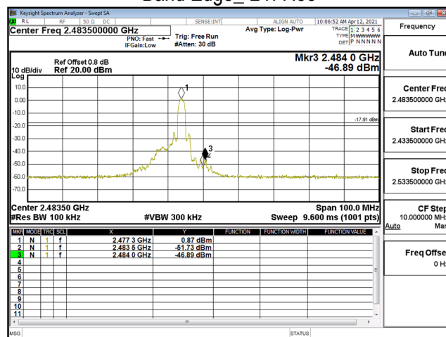
Band Edge _2477.35
