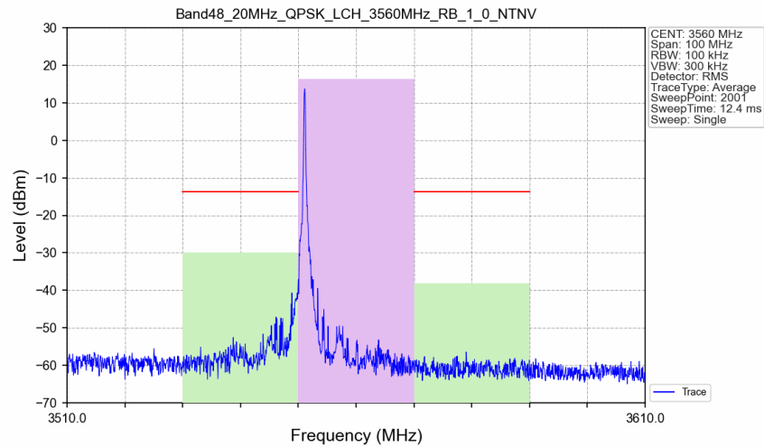
Band48_20MHz_QPSK_LCH_3560MHz_RB_1_0_NTNV
