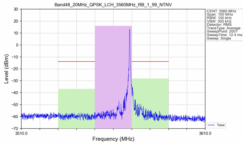
Band48_20MHz_QPSK_LCH_3560MHz_RB_1_99_NTNV
