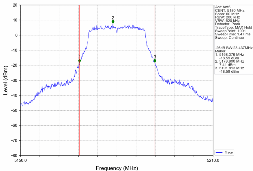
802.11n(HT20) LCH 5180MHz Ant5 NTN
