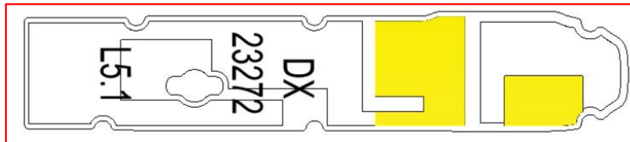
天线外观图
