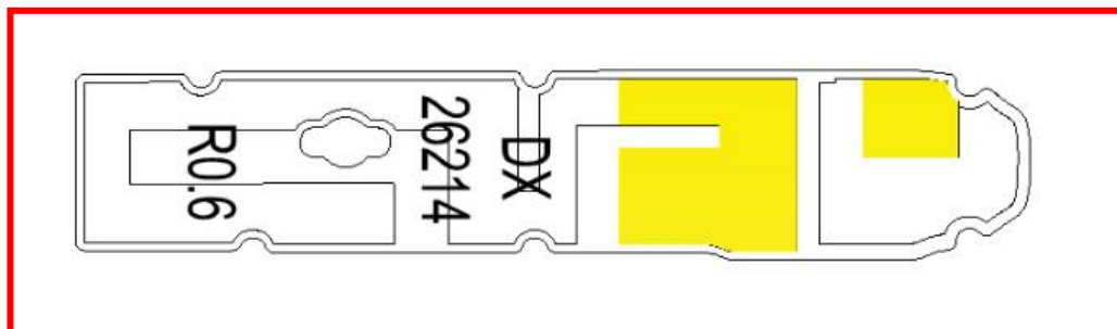
天线外观图
