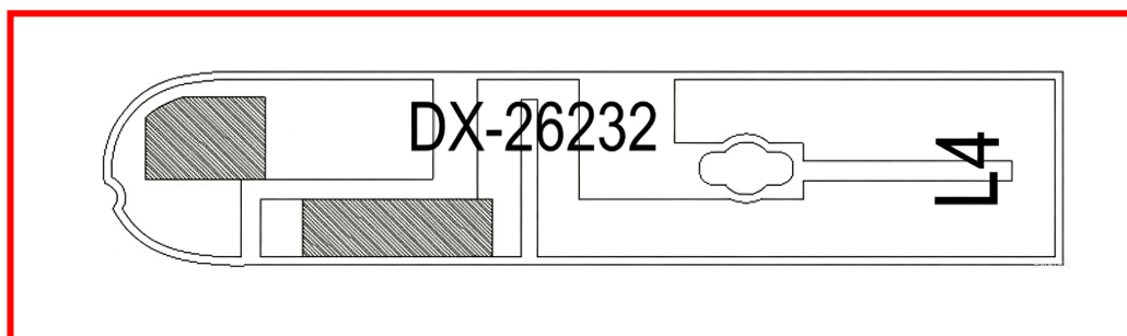
天线外观图
