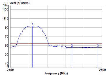
Antenna 2 11b_TX_CH_11_Horizontal-Avg
