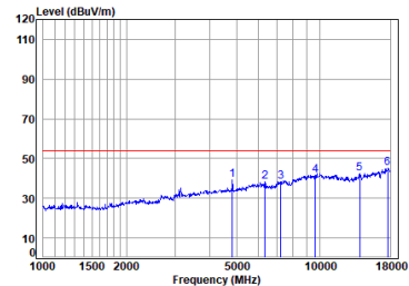
Antenna 2 11n_HT(20M)_TX_CH_01_Horizontal-Avg
