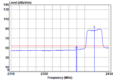
Antenna 2 11n_HT(20M)_TX_CH_01_Horizontal-Avg
