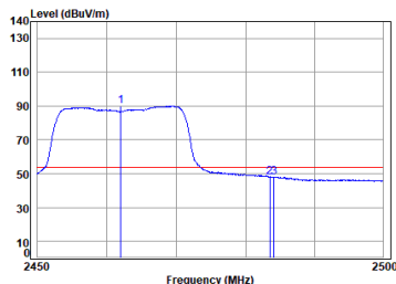
Antenna 1 11n_HT(20M)_TX_CH_11_Horizontal-Avg
