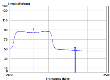
Antenna 2 11n_HT(20M)_TX_CH_11_Horizontal-Avg
