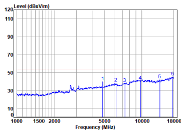
Antenna 2 11b_TX_CH_06_Horizontal-Avg
