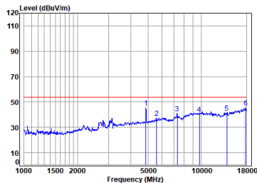
Antenna 2 11b_TX_CH_06_Vertical-Avg
