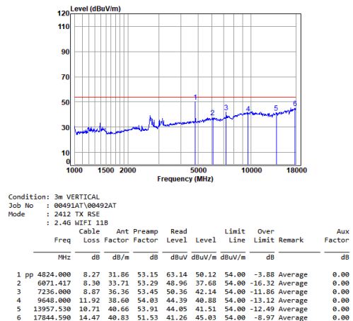
Antenna 1 11b_TX_CH_01_Vertical-Avg
