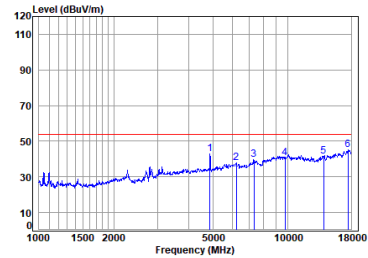
Antenna 2 11n_HT(20M)_TX_CH_06_Vertical-Avg
