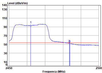
Antenna 2 11n_HT(20M)_TX_CH_11_Vertical-Avg
