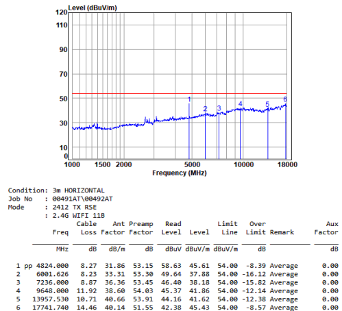
Antenna 1 11b_TX_CH_01_Horizontal-Avg
