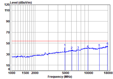
Antenna 2 11n_HT(20M)_TX_CH_11_Horizontal-Avg
