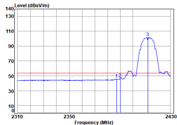
Antenna 2 11b_TX_CH_01_Vertical-Avg
