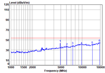
Antenna 2 11n_HT(20M)_TX_CH_11_Vertical-Avg
