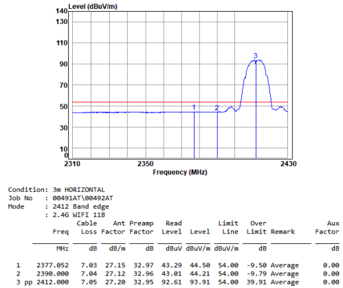
Antenna 1 11b_TX_CH_01_Horizontal-Avg
