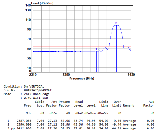
Antenna 1 11b_TX_CH_01_Vertical-Avg
