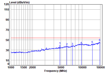
Antenna 2 11n_HT(20M)_TX_CH_06_Horizontal-Avg
