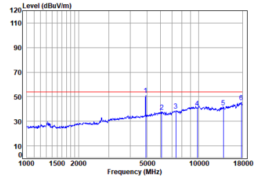
Antenna 1 11n_HT(20M)_TX_CH_11_Horizontal-Avg
