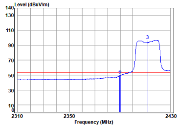
Antenna 2 11n_HT(20M)_TX_CH_01_Vertical-Avg
