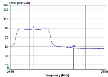
Antenna 2 11g_TX_CH_11_Horizontal-Avg
