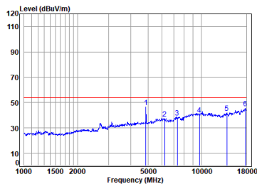
Antenna 1 11b_TX_CH_06_Horizontal-Avg
