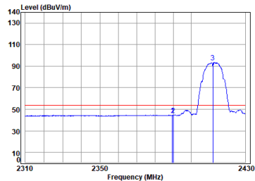
Antenna 2 11b_TX_CH_01_Horizontal-Avg
