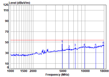
Antenna 2 11b_TX_CH_11_Vertical-Avg
