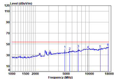
Antenna 2 11n_HT(20M)_TX_CH_01_Vertical-Avg
