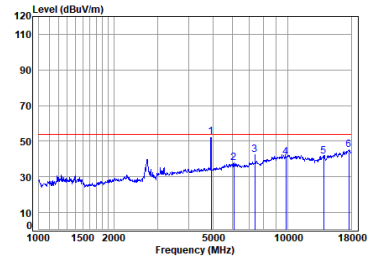
Antenna 1 11n_HT(20M)_TX_CH_11_Vertical-Avg
