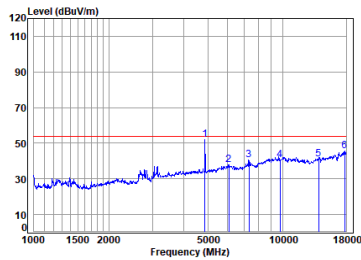
Antenna 1 11b_TX_CH_06_Vertical-Avg
