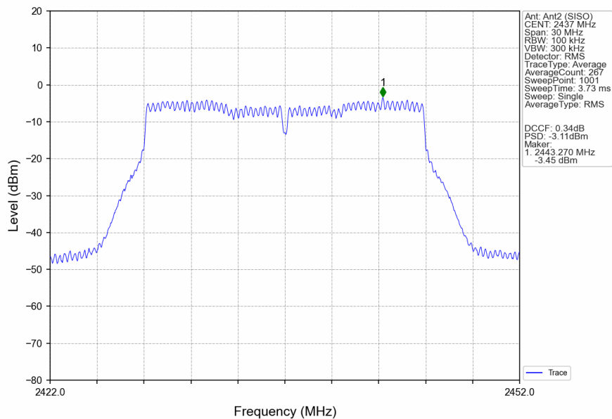
802.11n(HT20)_MCH_2437MHz_Ant2 (SISO)_NTNV
