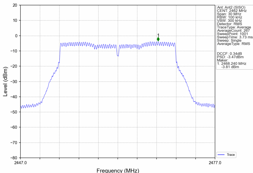
802.11n(HT20)_HCH_2462MHz_Ant2 (SISO)_NTNV
