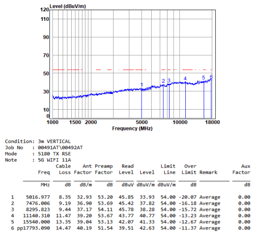
Antenna 1 11a_TX_CH_36_Vertical-Avg
