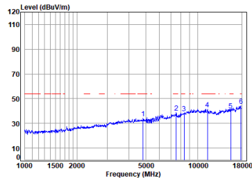
Antenna 2 11a_TX_CH_36_Horizontal-Avg
