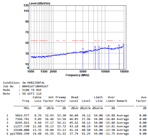
Antenna 1 11a_TX_CH_36_Horizontal-Avg
