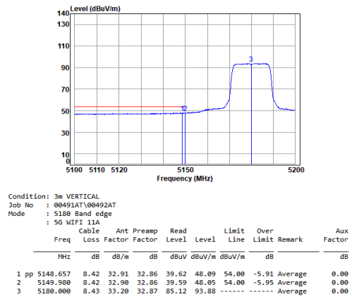
Antenna 1 11a_TX_CH_36_Vertical-Avg
