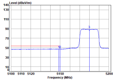
Antenna 2 11ac_VHT(20M)_TX_CH_36_Vertical-Avg
