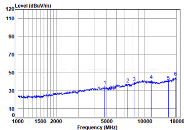
Antenna 2 11a_TX_CH_36_Vertical-Avg
