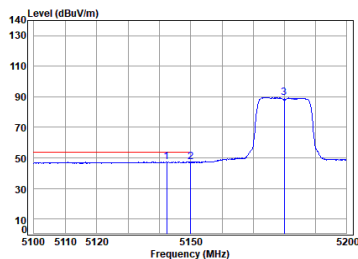
Antenna 2 11a_TX_CH_36_Vertical-Avg
