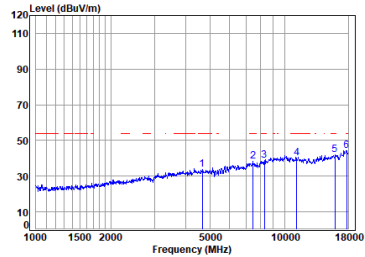
Antenna 1 11a_TX_CH_116_Horizontal-Avg
