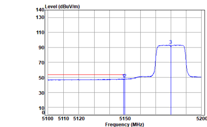
Antenna 1 11ac_VHT(20M)_TX_CH_36_Vertical-Avg
