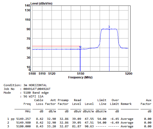
Antenna 1 11a_TX_CH_36_Horizontal-Avg
