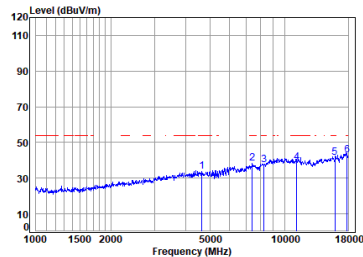
Antenna 2 11a_TX_CH_116_Horizontal-Avg
