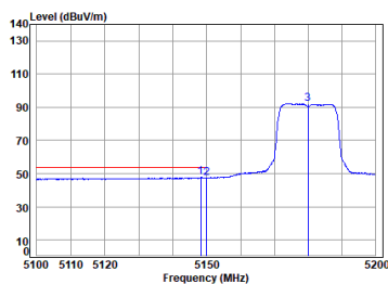
Antenna 2 11a_TX_CH_36_Horizontal-Avg
