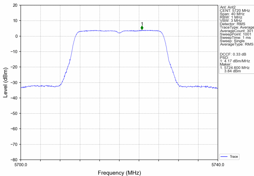
802.11n(HT20)_HCH_5720MHz_Ant2_NTNV
