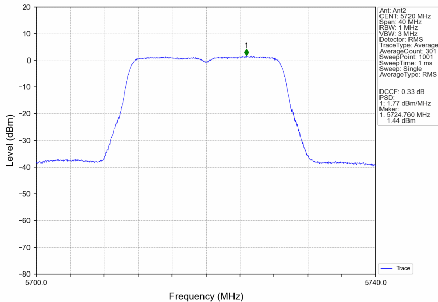
802.11ac(VHT20)_HCH_5720MHz_Ant2_NTNV
