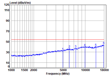
Antenna 2 BLE_2M_TX_CH_39_Vertical-Avg
