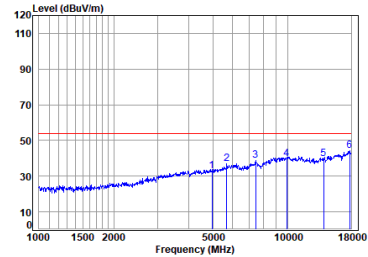
Antenna 1 BLE_2M_TX_CH_39_Horizontal-Avg
