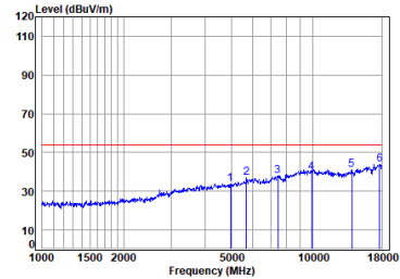
Antenna 2 BLE_1M_TX_CH_39_Horizontal-Avg
