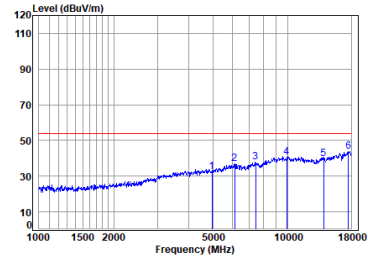
Antenna 2 BLE_2M_TX_CH_39_Horizontal-Avg
