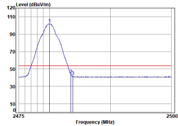
Antenna 2 BLE_2M_TX_CH_39_Vertical-Avg
