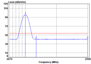
Antenna 2 BLE_1M_TX_CH_39_Horizontal-Avg
