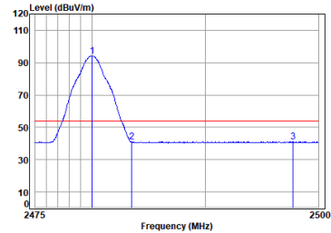
Antenna 2 BLE_2M_TX_CH_39_Horizontal-Avg
