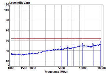
Antenna 1 BLE_2M_TX_CH_39_Vertical-Avg
