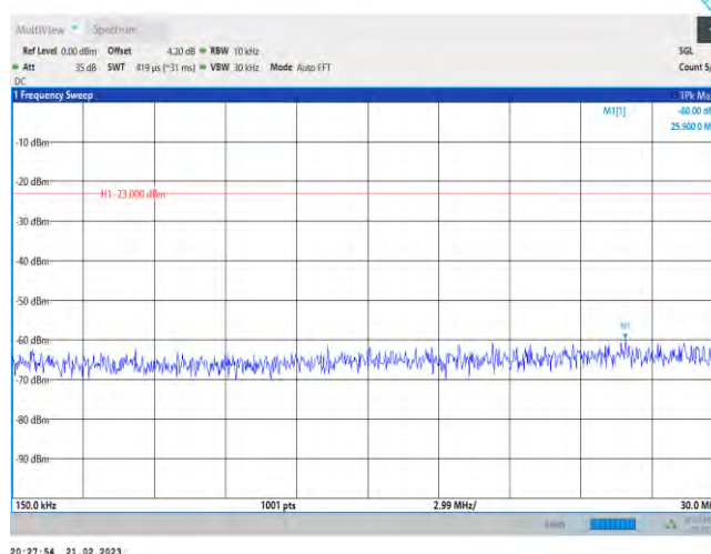
Band4-20MHz-QPSK-20050-1RB#0-Range2:0.15~30MHz
