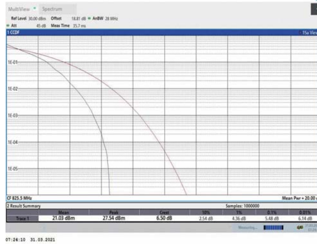
Band5-3MHz-QPSK-20415-1RB#0
