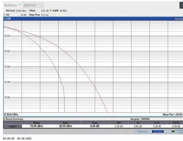
Band5-10MHz-QPSK-20450-1RB#0
