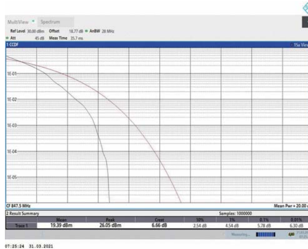
Band5-3MHz-QPSK-20635-1RB#0
