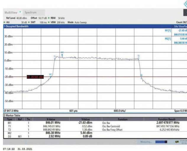
Band5-3MHz-QPSK-20635-15RB#0-2.697
