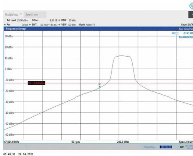
Band5-3MHz-QPSK-20415-1RB#0
