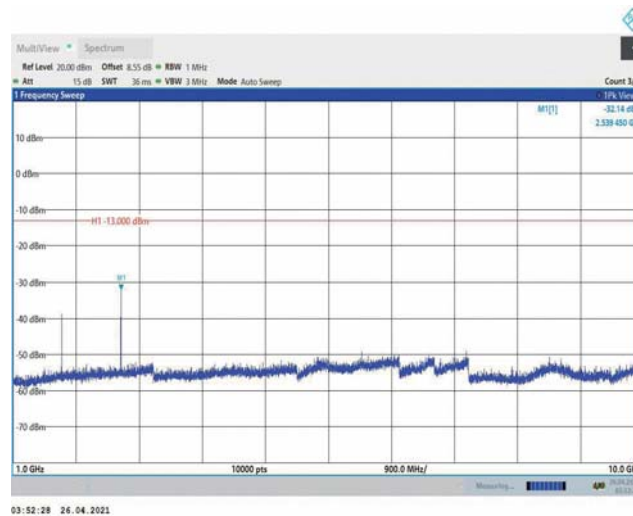
Band5-3MHz-QPSK-20635-1RB#0-Range2:1000~10000MHz
