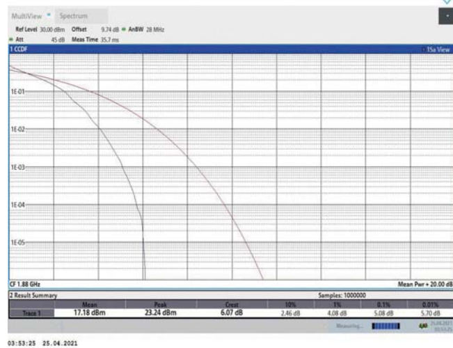
Band2-3MHz-QPSK-18900-1RB#0
