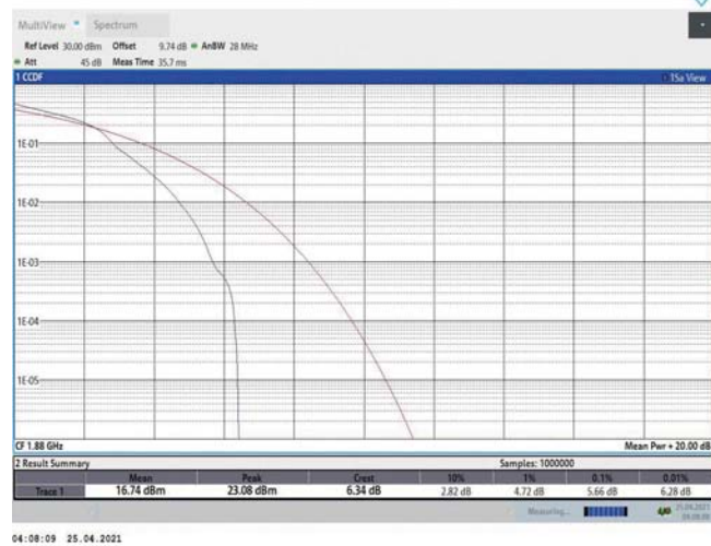
Band2-5MHz-16QAM-18900-1RB#0
