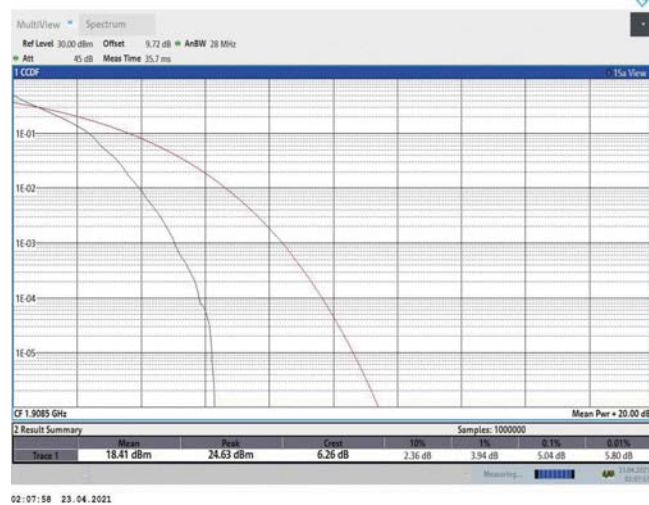
Band2-3MHz-QPSK-19185-1RB#0
