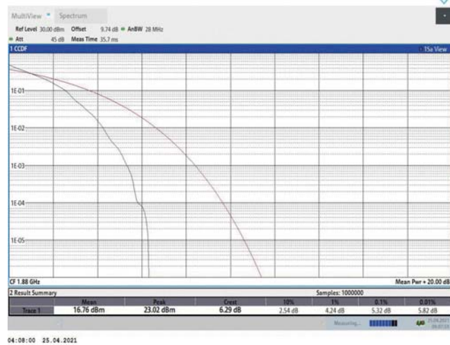
Band2-5MHz-QPSK-18900-1RB#0
