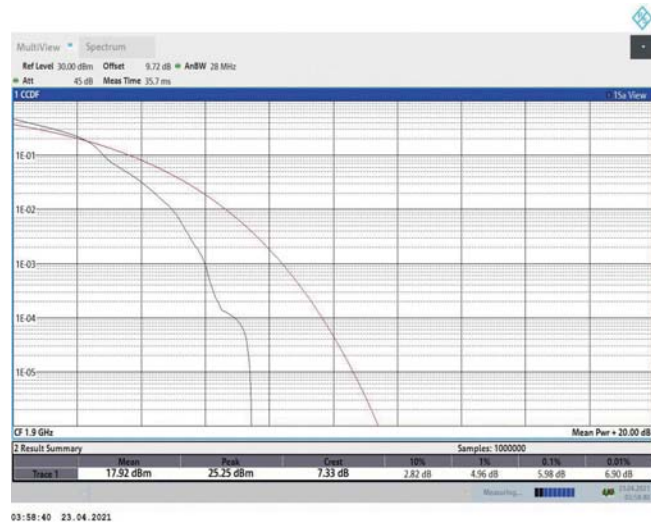
Band2-20MHz-16QAM-19100-1RB#0
