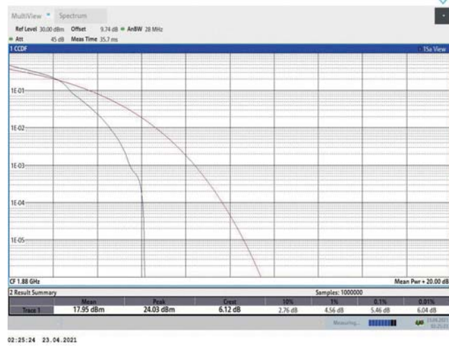
Band2-5MHz-16QAM-18900-1RB#0
