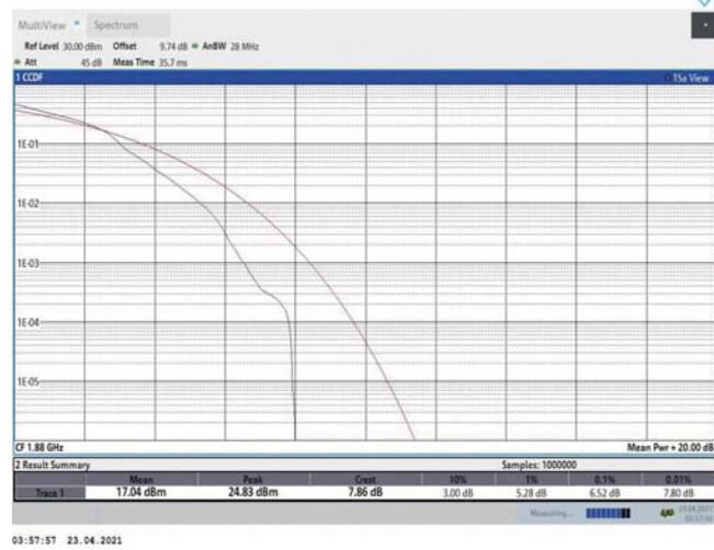
Band2-20MHz-16QAM-18900-1RB#0
