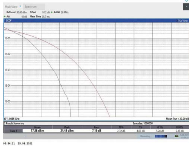
Band2-3MHz-QPSK-19185-15RB#0
