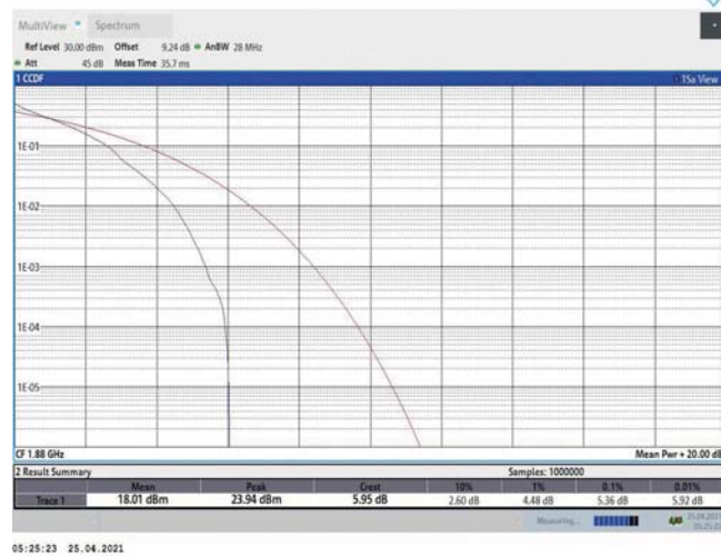
Band2-20MHz-QPSK-18900-1RB#0
