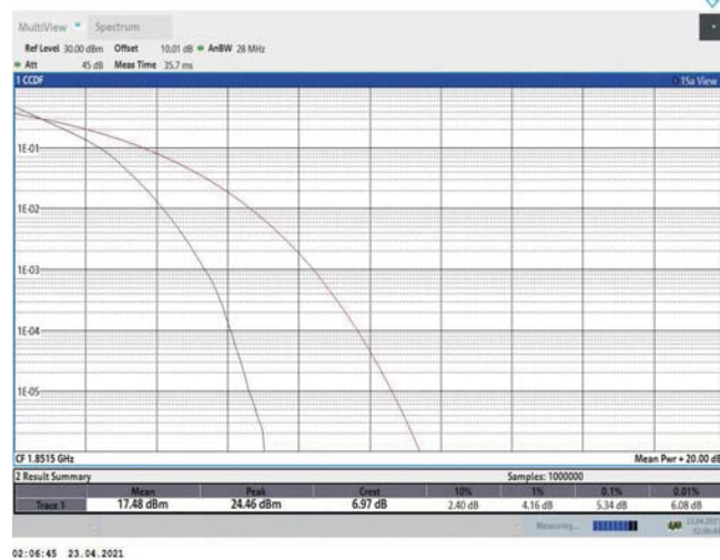
Band2-3MHz-QPSK-18615-15RB#0
