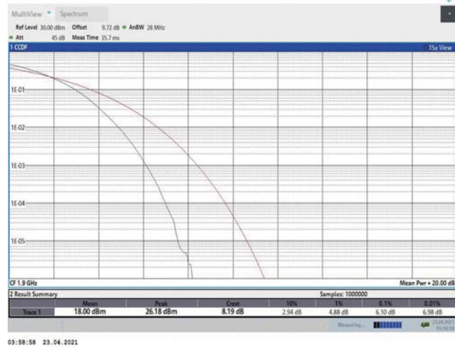
Band2-20MHz-16QAM-19100-100RB#0
