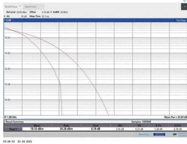
Band2-10MHz-QPSK-18900-1RB#0
