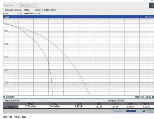
Band2-20MHz-QPSK-18900-1RB#0
