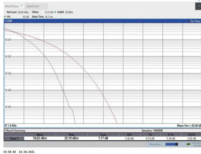
Band2-20MHz-QPSK-19100-100RB#0
