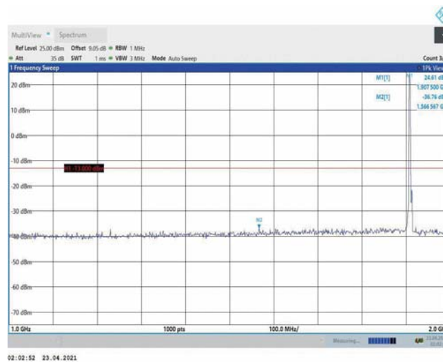
Band2-3MHz-16QAM-19185-1RB#0-Range2:1000~2000MHz
