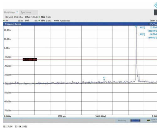
Band2-10MHz-QPSK-18650-1RB#0-Range2:1000~2000MHz
