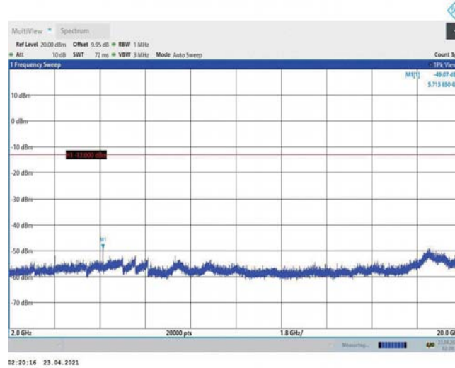
Band2-5MHz-QPSK-19175-1RB#0-Range3:2000~20000MHz
