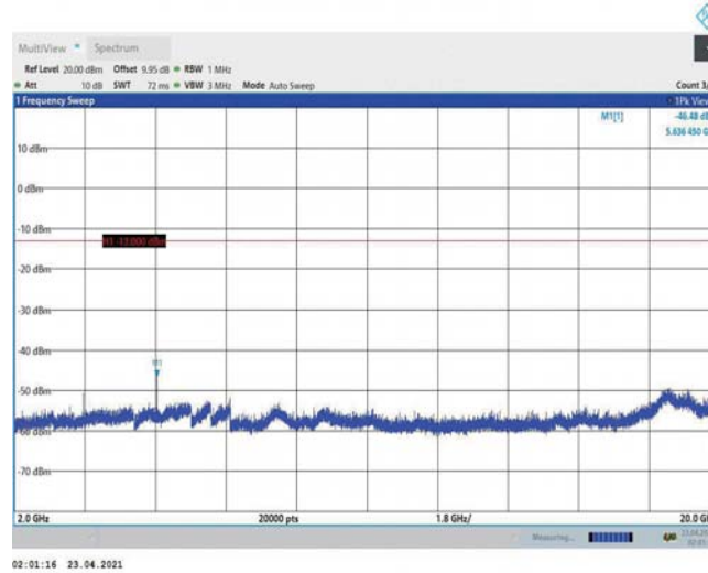
Band2-3MHz-QPSK-18900-1RB#0-Range3:2000~20000MHz
