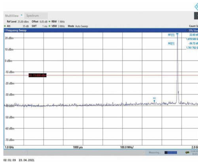
Band2-3MHz-QPSK-18900-1RB#0-Range2:1000~2000MHz
