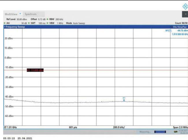
Band2-20MHz-QPSK-19100-1RB#0
