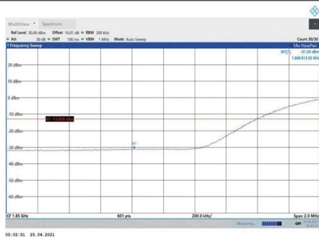
Band2-20MHz-16QAM-18700-100RB#0
