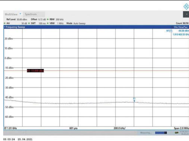
Band2-20MHz-16QAM-19100-1RB#0
