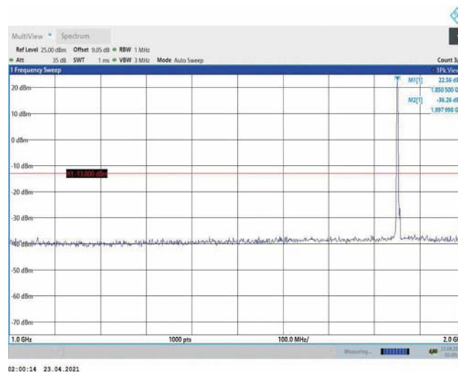
Band2-3MHz-16QAM-18615-1RB#0-Range2:1000~2000MHz
