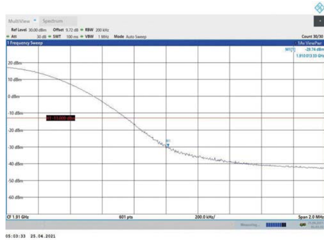
Band2-20MHz-QPSK-19100-1RB#99
