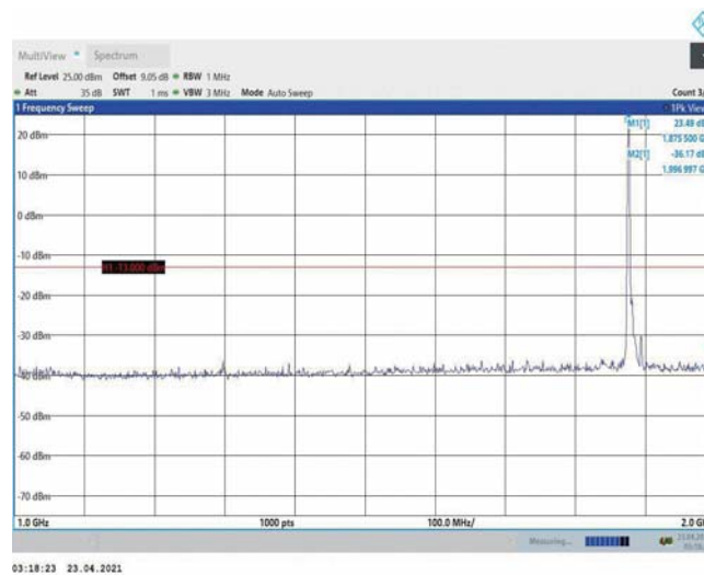
Band2-10MHz-QPSK-18900-1RB#0-Range2:1000~2000MHz
