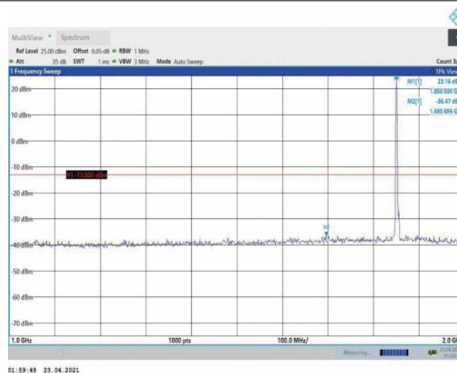
Band2-3MHz-QPSK-18615-1RB#0-Range2:1000~2000MHz
