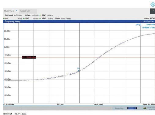
Band2-20MHz-16QAM-18700-1RB#0
