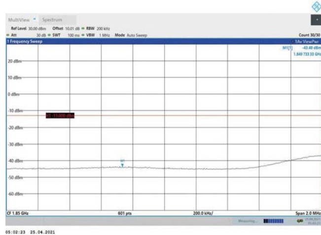
Band2-20MHz-QPSK-18700-1RB#99
