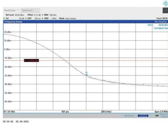
Band2-20MHz-16QAM-19100-1RB#99
