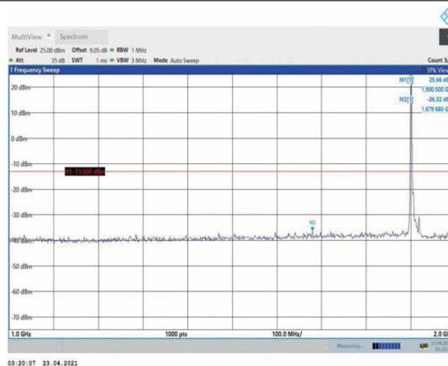
Band2-10MHz-16QAM-19150-1RB#0-Range2:1000~2000MHz
