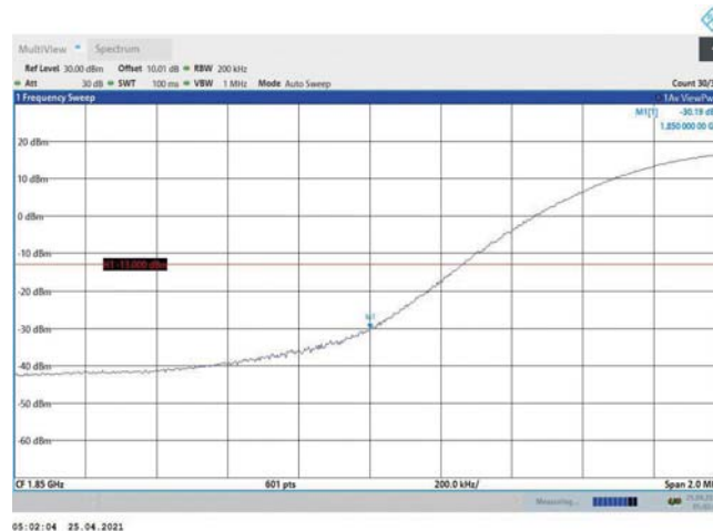
Band2-20MHz-QPSK-18700-1RB#0
