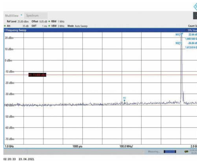
Band2-5MHz-16QAM-19175-1RB#0-Range2:1000~2000MHz
