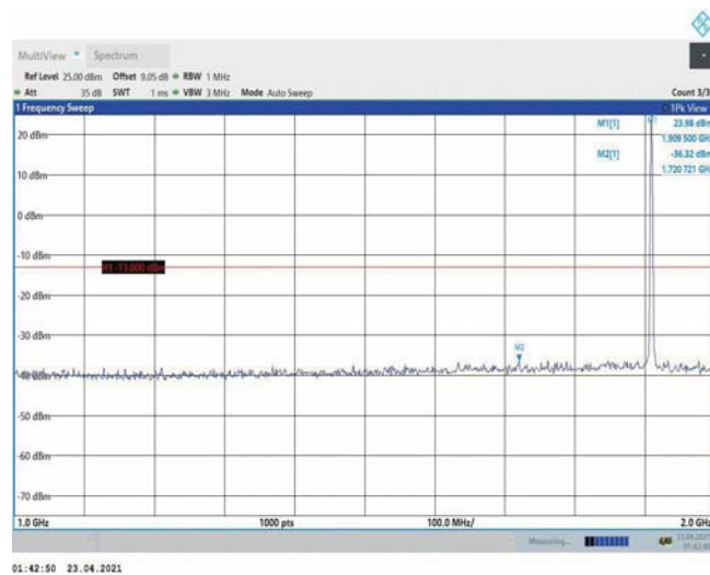
Band2-1.4MHz-QPSK-19193-1RB#0-Range2:1000~2000MHz
