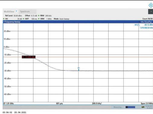
Band2-20MHz-16QAM-19100-100RB#0
