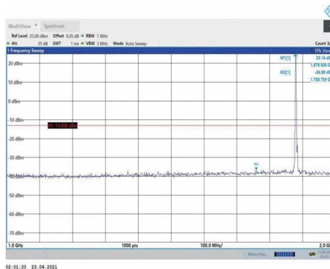
Band2-3MHz-16QAM-18900-1RB#0-Range2:1000~2000MHz
