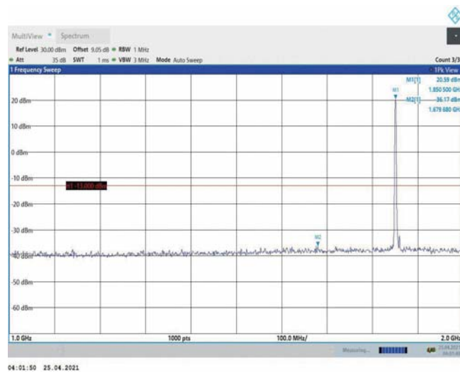
Band2-5MHz-QPSK-18625-1RB#0-Range2:1000~2000MHz
