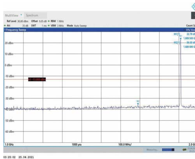
Band2-1.4MHz-QPSK-19193-1RB#0-Range2:1000~2000MHz
