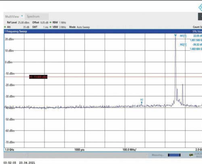
Band2-20MHz-16QAM-18700-1RB#0-Range2:1000~2000MHz
