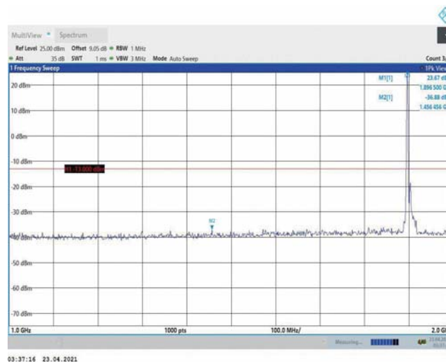
Band2-15MHz-QPSK-19125-1RB#0-Range2:1000~2000MHz
