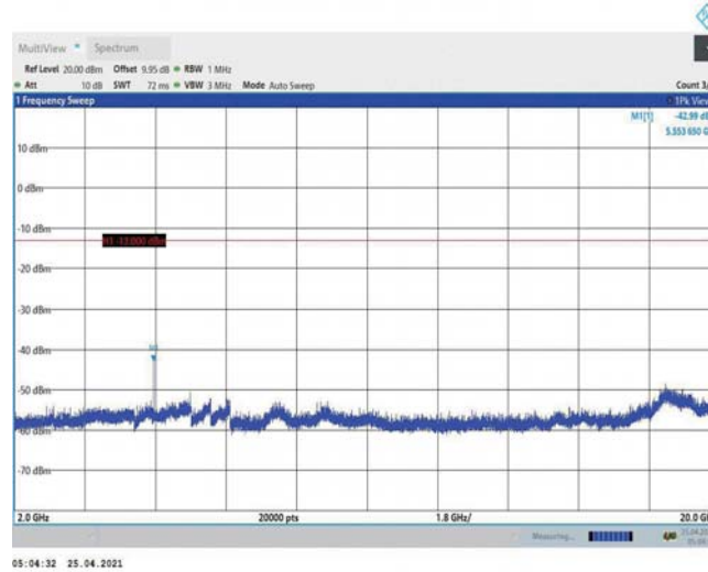
Band2-20MHz-QPSK-18700-1RB#0-Range3:2000~20000MHz
