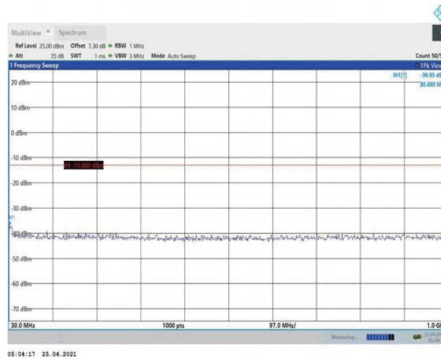
Band2-20MHz-QPSK-18700-1RB#0-Range1:30~1000MHz
