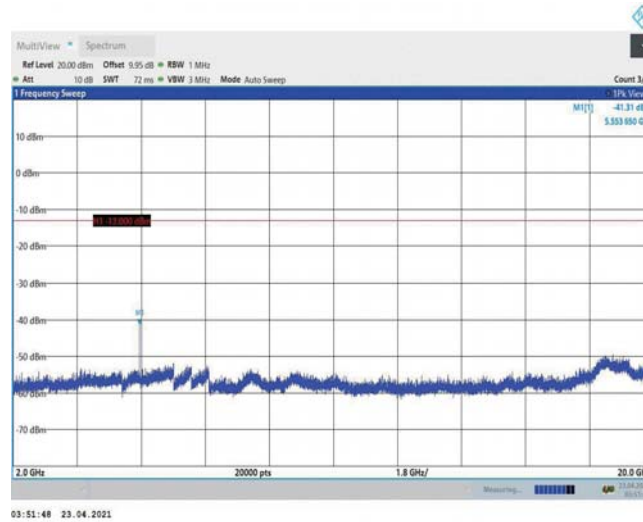
Band2-20MHz-QPSK-18700-1RB#0-Range3:2000~20000MHz
