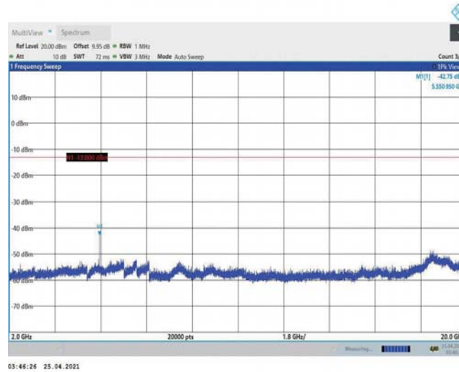
Band2-3MHz-QPSK-18615-1RB#0-Range3:2000~20000MHz
