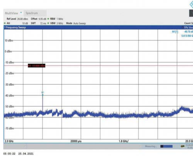
Band2-20MHz-QPSK-18900-1RB#0-Range3:2000~20000MHz
