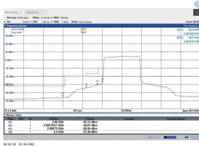
Band7-10MHz-QPSK-20800-50RB#0
