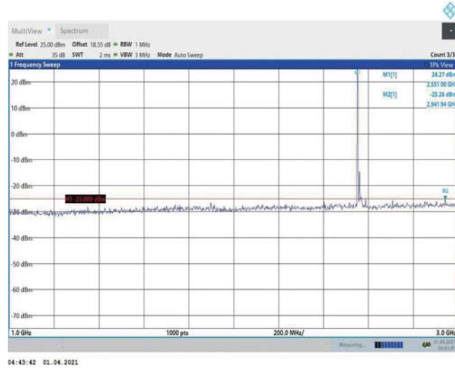
Band7-20MHz-QPSK-21350-1RB#0-Range2:1000~3000MHz
