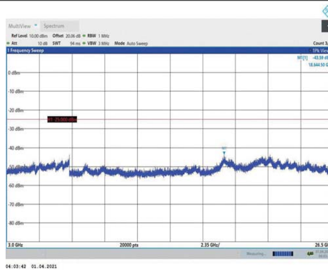
Band7-10MHz-QPSK-20800-1RB#0-Range3:3000~26500MHz
