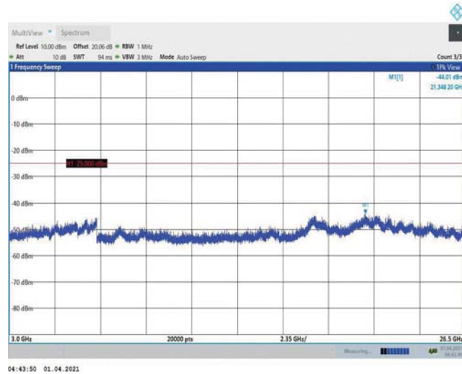
Band7-20MHz-QPSK-21350-1RB#0-Range3:3000~26500MHz
