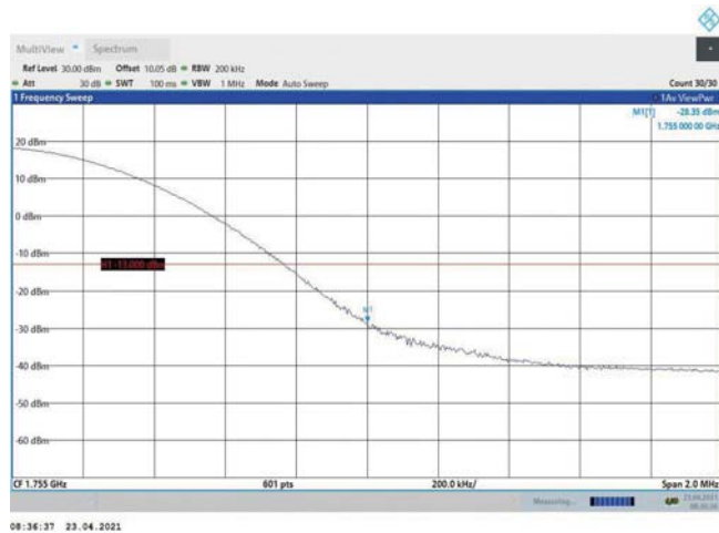
Band4-20MHz-QPSK-20300-1RB#99
