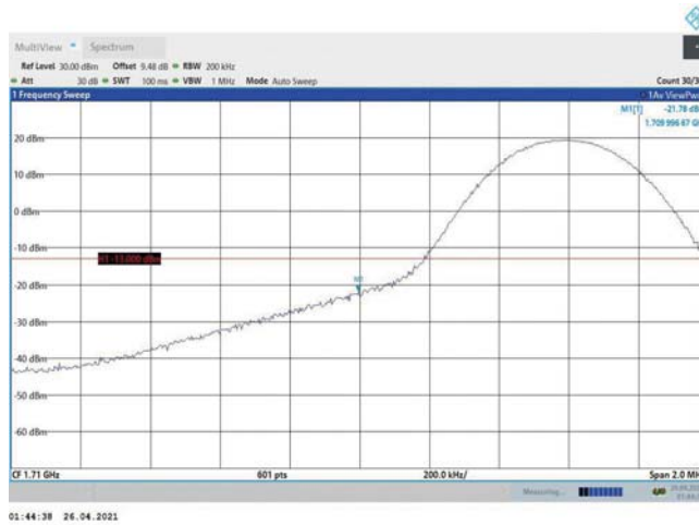
Band4-10MHz-QPSK-20000-1RB#0
