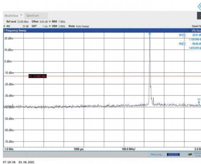
Band4-10MHz-QPSK-20175-1RB#0-Range2:1000~2000MHz
