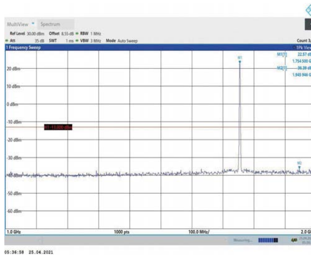
Band4-1.4MHz-QPSK-20393-1RB#0-Range2:1000~2000MHz
