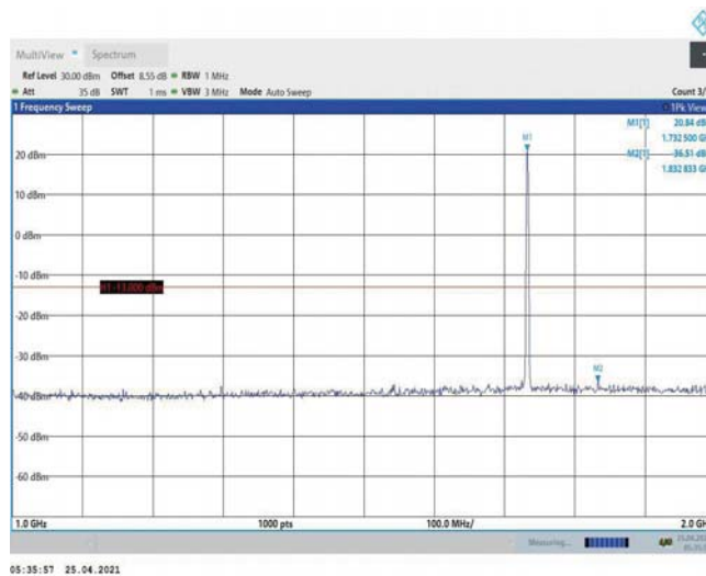
Band4-1.4MHz-QPSK-20175-1RB#0-Range2:1000~2000MHz
