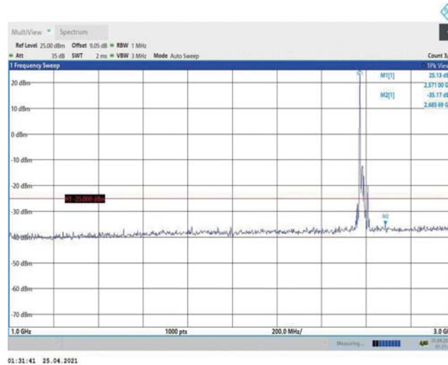
Band38-20MHz-16QAM-37850-1RB#0-Range2:1000~3000MHz
