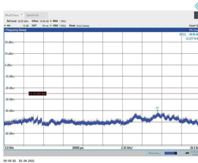
Band38-5MHz-QPSK-38225-1RB#0-Range3:3000~26500MHz
