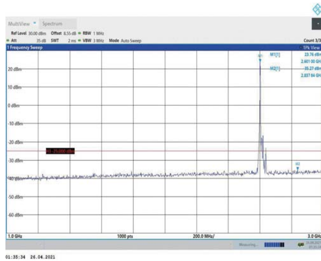
Band38-20MHz-QPSK-38150-1RB#0-Range2:1000~3000MHz
