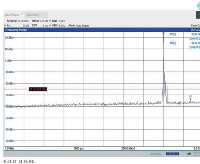
Band38-20MHz-QPSK-38150-1RB#0-Range2:1000~3000MHz
