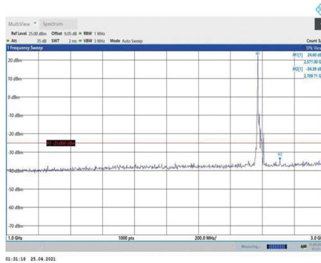
Band38-20MHz-QPSK-37850-1RB#0-Range2:1000~3000MHz
