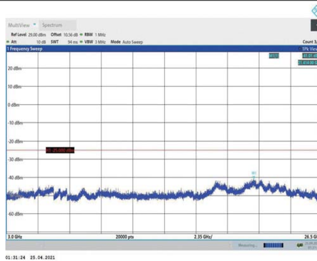
Band38-20MHz-QPSK-37850-1RB#0-Range3:3000~26500MHz
