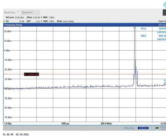
Band38-20MHz-QPSK-38000-1RB#0-Range2:1000~3000MHz
