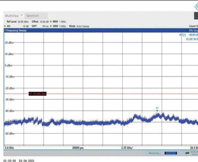
Band38-20MHz-QPSK-37850-1RB#0-Range3:3000~26500MHz
