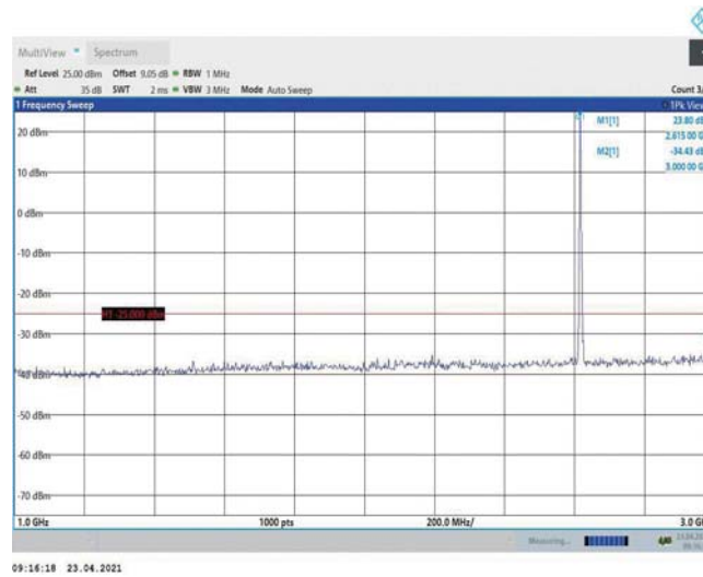
Band38-5MHz-QPSK-38225-1RB#0-Range2:1000~3000MHz
