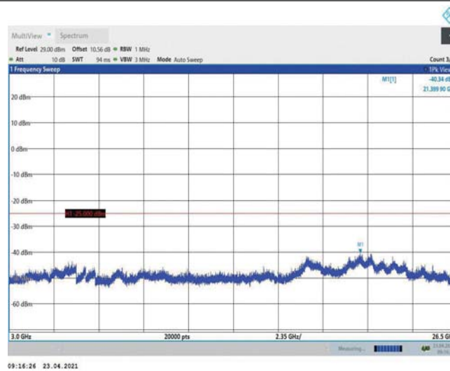
Band38-5MHz-QPSK-38225-1RB#0-Range3:3000~26500MHz
