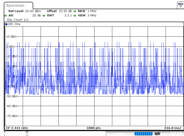
2EDR_DH1_Hopping
