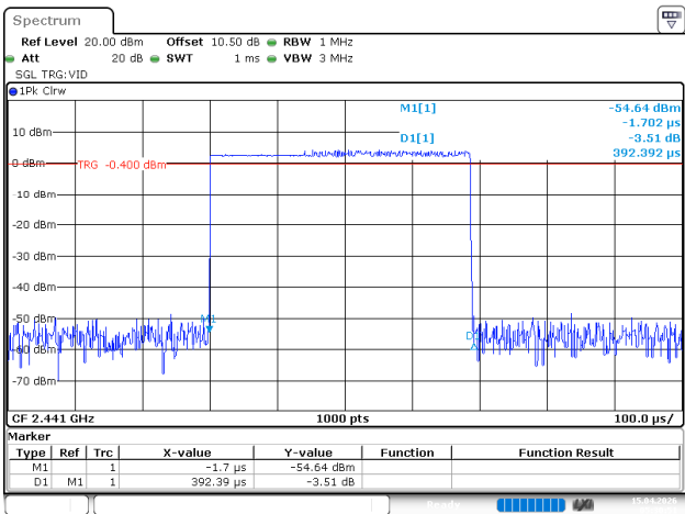
2EDR_DH1_Hopping
