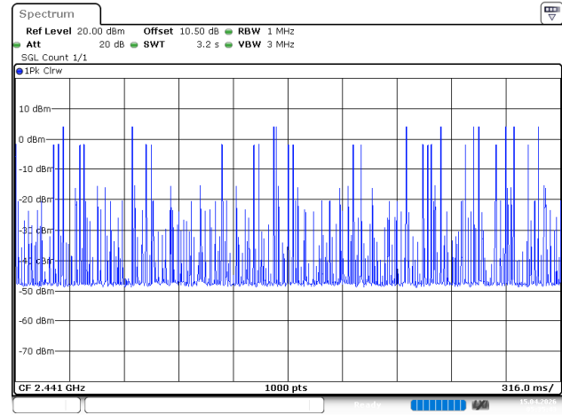
2EDR_DH5_Hopping
