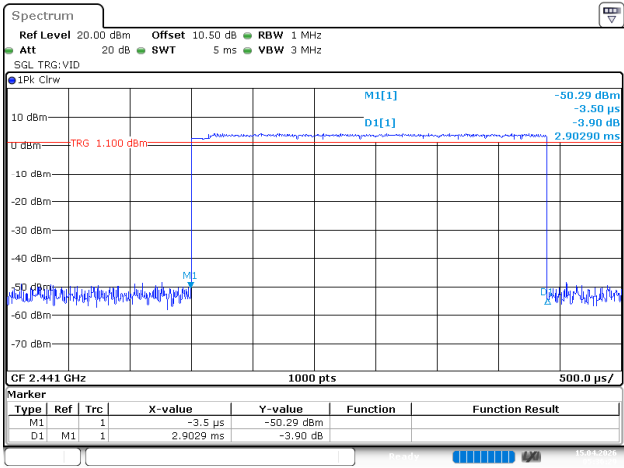
2EDR_DH5_Hopping
