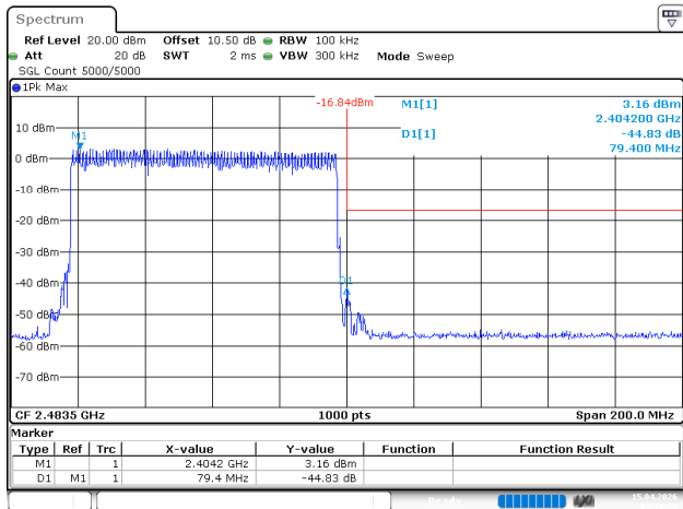
3EDR_DH1_Hopping_Upper
