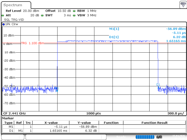
2EDR_DH3_Hopping
