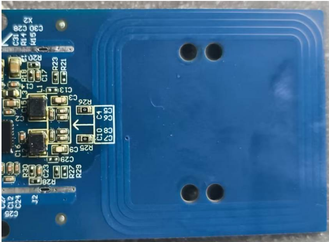
NFC Antenna
