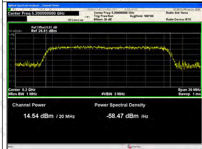
802.11ax(HE20)-5200
