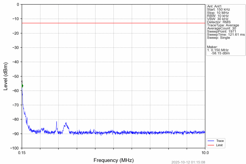
Band5_3MHz_QPSK_HCH_847.5MHz_RB_1_0_NTNV
