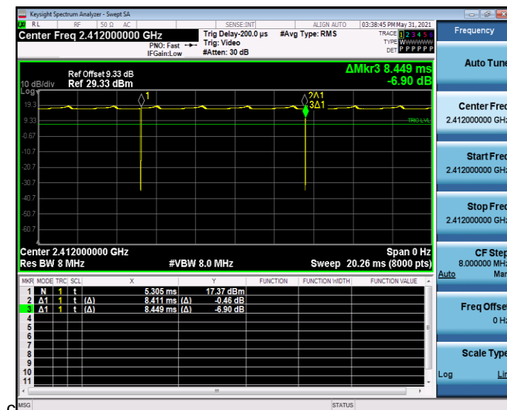
11B_Ant1_2412
