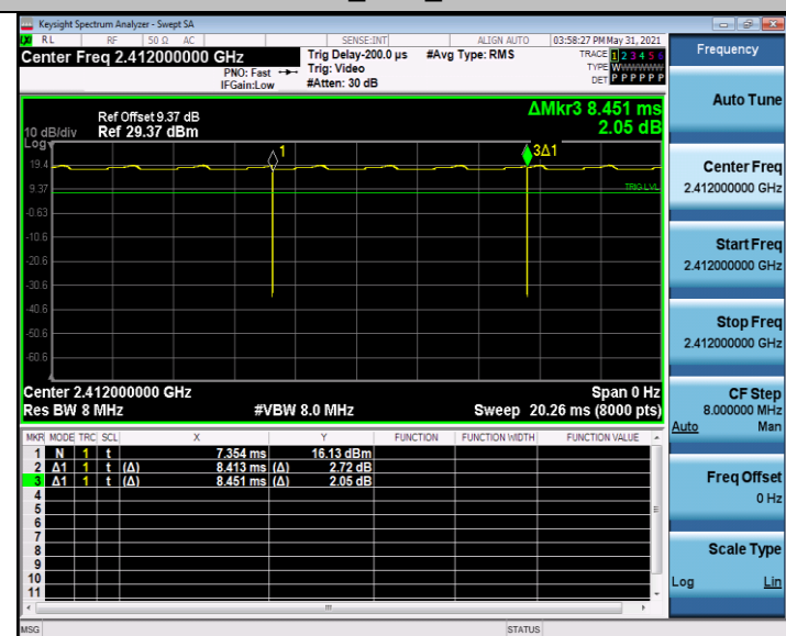
11B_Ant2_2412
