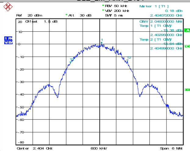
BLE_2M_Ant1_2404
