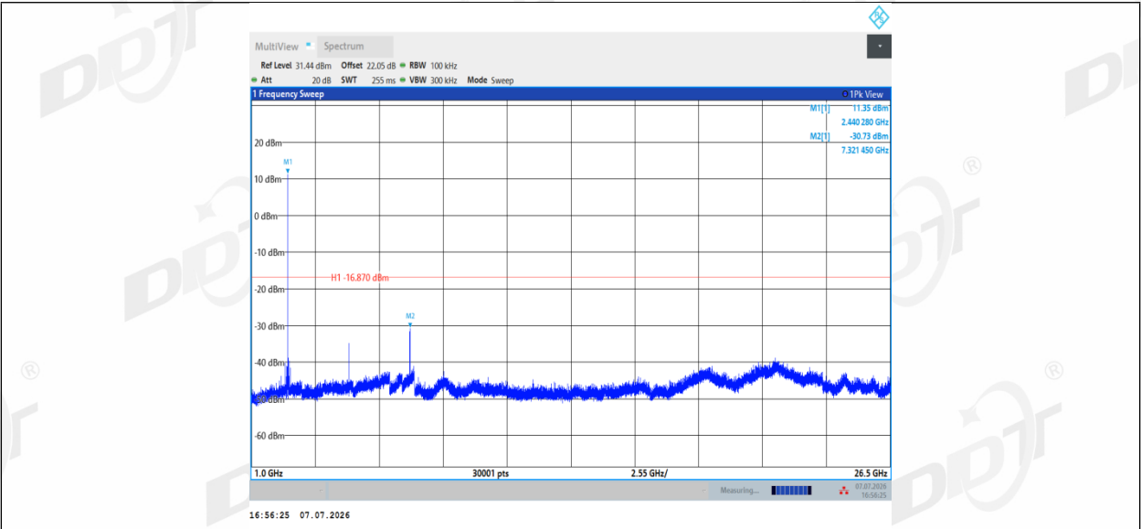
BLE 2M_Ant1_2478_0-Reference
