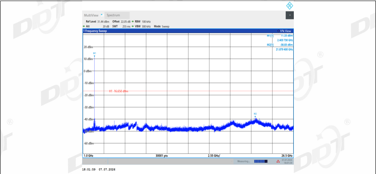
BLE 2M_Ant1_2440_0~Reference
