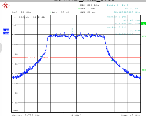
20 MHZ Ant1 5785
