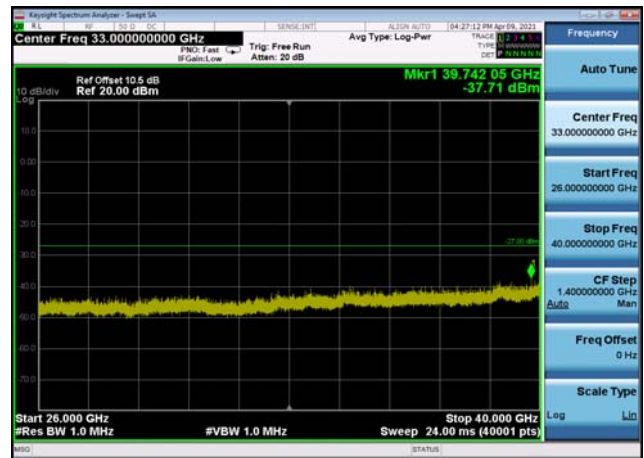
U-NII-1 ,Plot 2,26000MHz~40000MHz-802 .11n(20MHz),5240MHz,Ant0
