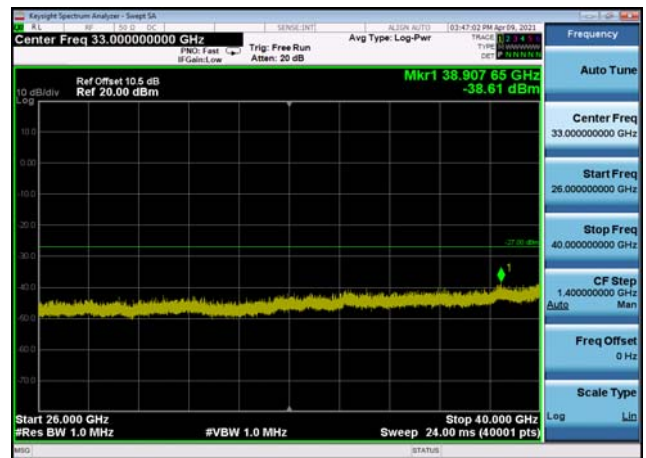
U-NII-1 ,Plot 2,26000MHz~40000MHz-802 .11n(20MHz),5180MHz,Ant1
