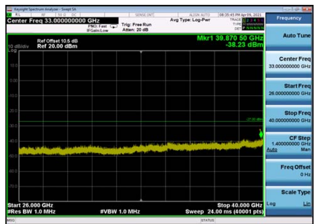
U-NII-1 ,Plot 2,26000MHz~40000MHz-802 .11a(20MHz),5240MHz,Ant0
