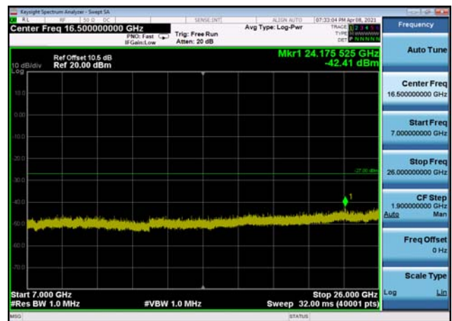
U-NII-3 ,Plot 4,7000MHz~26000MHz-802. 11ac(40MHz),5755MHz,Ant1
