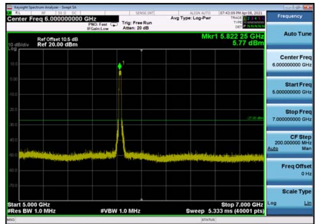
U-NII-3 ,Plot 3,5000MHz~7000MHz-802.1 1ac(40MHz),5795MHz,Ant1
