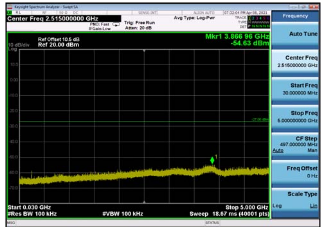
U-NII-3 ,Plot 2,30MHz~5000MHz-802.11a c(40MHz),5755MHz,Ant1
