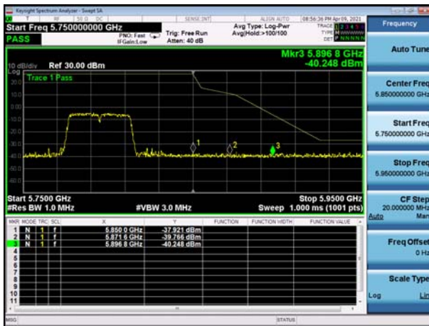
U-NII-3 ,Plot 1,Band Edge-802.11ac(40 MHz),5755MHz,Ant0
