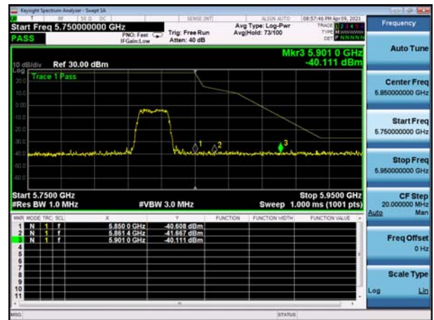
U-NII-3 ,Plot 1,Band Edge-802.11ac(80 MHz),5775MHz,Ant0 right edge
