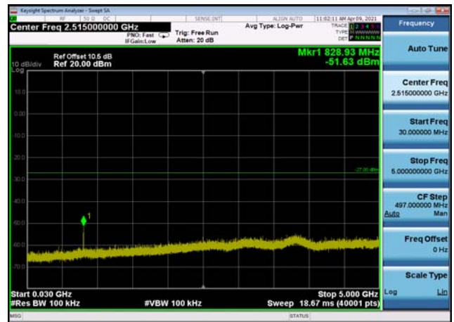
U-NII-3 ,Plot 2,30MHz~5000MHz-802.11a c(80MHz),5775MHz,Ant0
