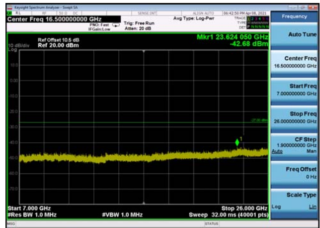
U-NII-3 ,Plot 4,7000MHz~26000MHz-802. 11ac(20MHz),5785MHz,Ant1
