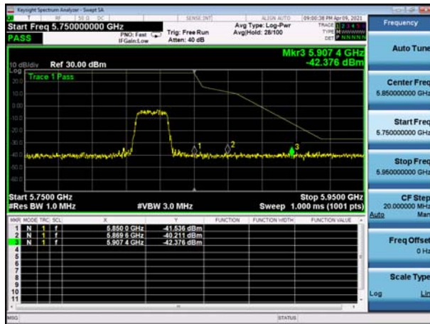
U-NII-3 ,Plot 1,Band Edge-802.11ac(40 MHz),5795MHz,Ant1
