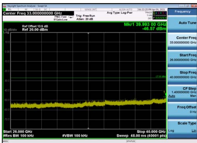
U-NII-3 ,Plot 2,26000MHz~40000MHz-802 .11ac(20MHz),5825MHz,Ant1
