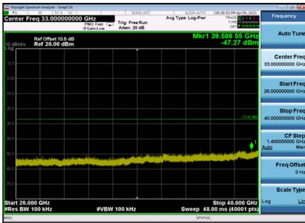
U-NII-3 ,Plot 2,26000MHz~40000MHz-802 .11ac(40MHz),5795MHz,Ant0
