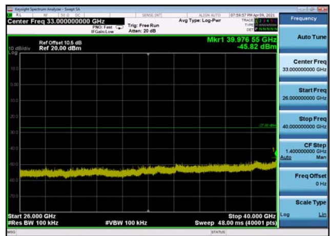
U-NII-3 ,Plot 2,26000MHz~40000MHz-802 .11ac(40MHz),5755MHz,Ant0
