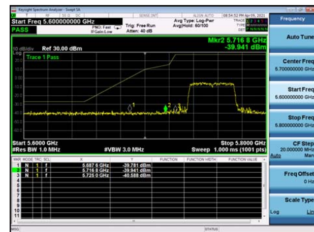
U-NII-3 ,Plot 1,Band Edge-802.11n(40M Hz),5755MHz,Ant0
