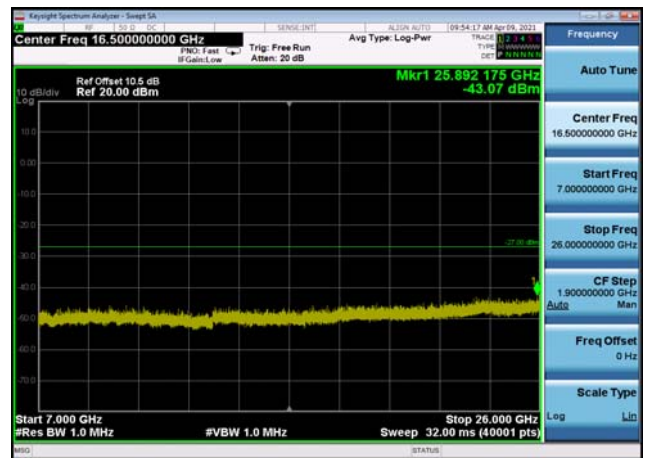
U-NII-3 ,Plot 4,7000MHz~26000MHz-802. 11ac(20MHz),5785MHz,Ant0
