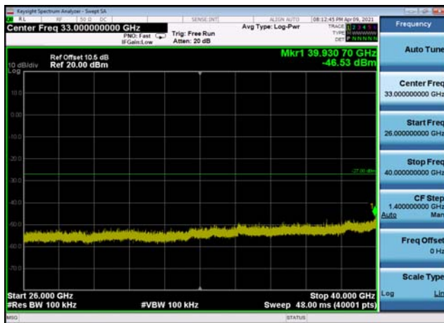
U-NII-3 ,Plot 2,26000MHz~40000MHz-802 .11ac(20MHz),5745MHz,Ant0
