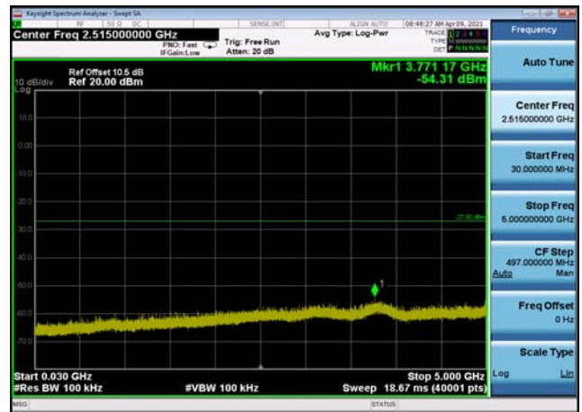
U-NII-3 ,Plot 2,30MHz~5000MHz-802.11a (20MHz),5825MHz,Ant0
