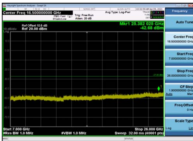
U-NII-3 ,Plot 4,7000MHz~26000MHz-802. 11n(40MHz),5755MHz,Ant0
