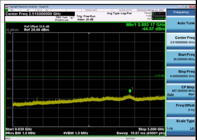
U-NII-1 ,Plot 2,30MHz~5000MHz-802.11 ax (20MHz),5180MHz,Ant1
