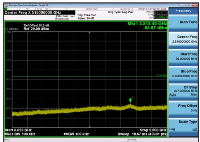
U-NII-3 ,Plot 2,30MHz~5000MHz-802.11a c(20MHz),5785MHz,Ant0
