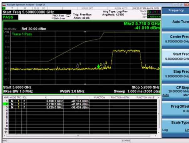
U-NII-3 ,Plot 1,Band Edge-802.11ac(80 MHz),5775MHz,Ant0 left edge
