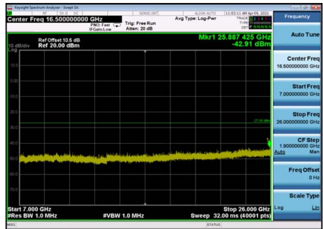
U-NII-3 ,Plot 4,7000MHz~26000MHz-802. 11ac(80MHz),5775MHz,Ant0
