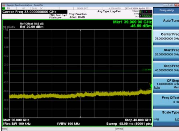
U-NII-3 ,Plot 2,26000MHz~40000MHz-802 .11ac(80MHz),5775MHz,Ant0
