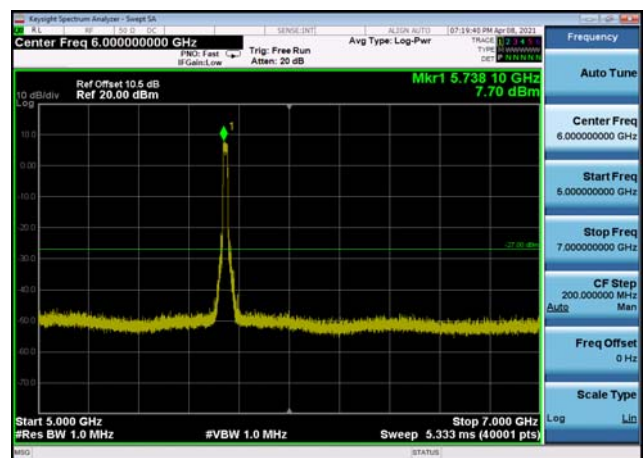
U-NII-3 ,Plot 3,5000MHz~7000MHz-802.1 1ac(20MHz),5745MHz,Ant1
