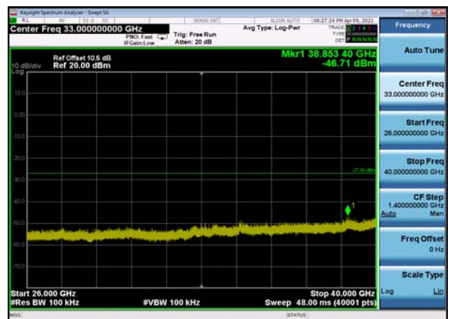
U-NII-3 ,Plot 2,26000MHz~40000MHz-802 .11n(20MHz),5825MHz,Ant0
