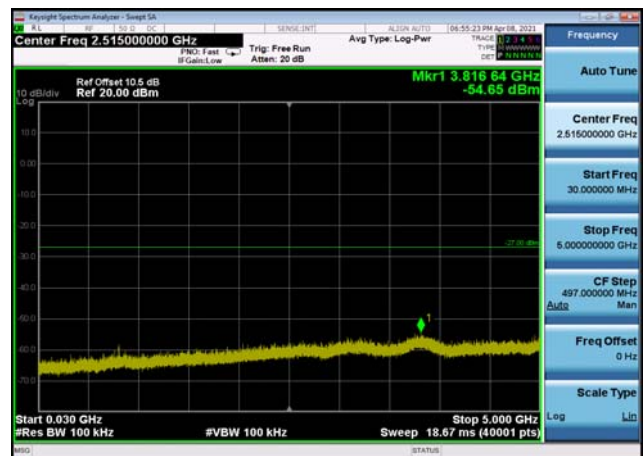
U-NII-3 ,Plot 2,30MHz~5000MHz-802.11n (20MHz),5825MHz,Ant1
