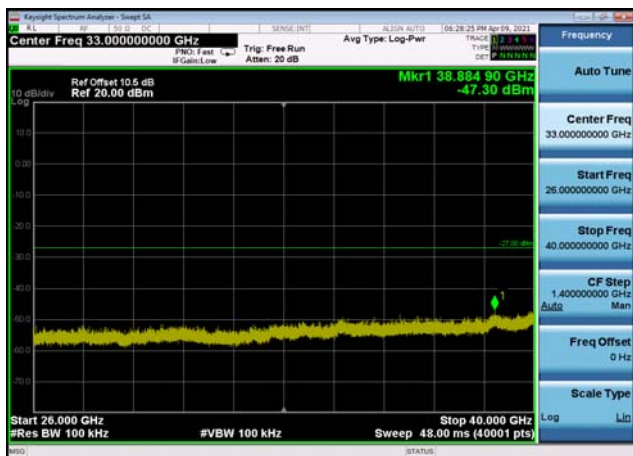
U-NII-3 ,Plot 2,26000MHz~40000MHz-802 .11ac(20MHz),5745MHz,Ant1
