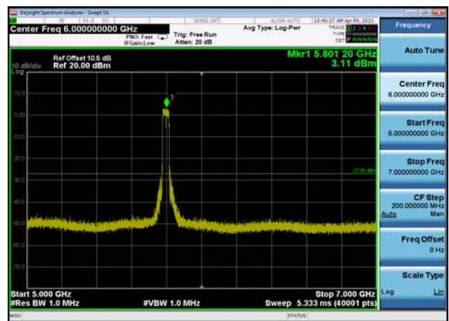
U-NII-3 ,Plot 3,5000MHz~7000MHz-802.1 1n(40MHz),5795MHz,Ant0
