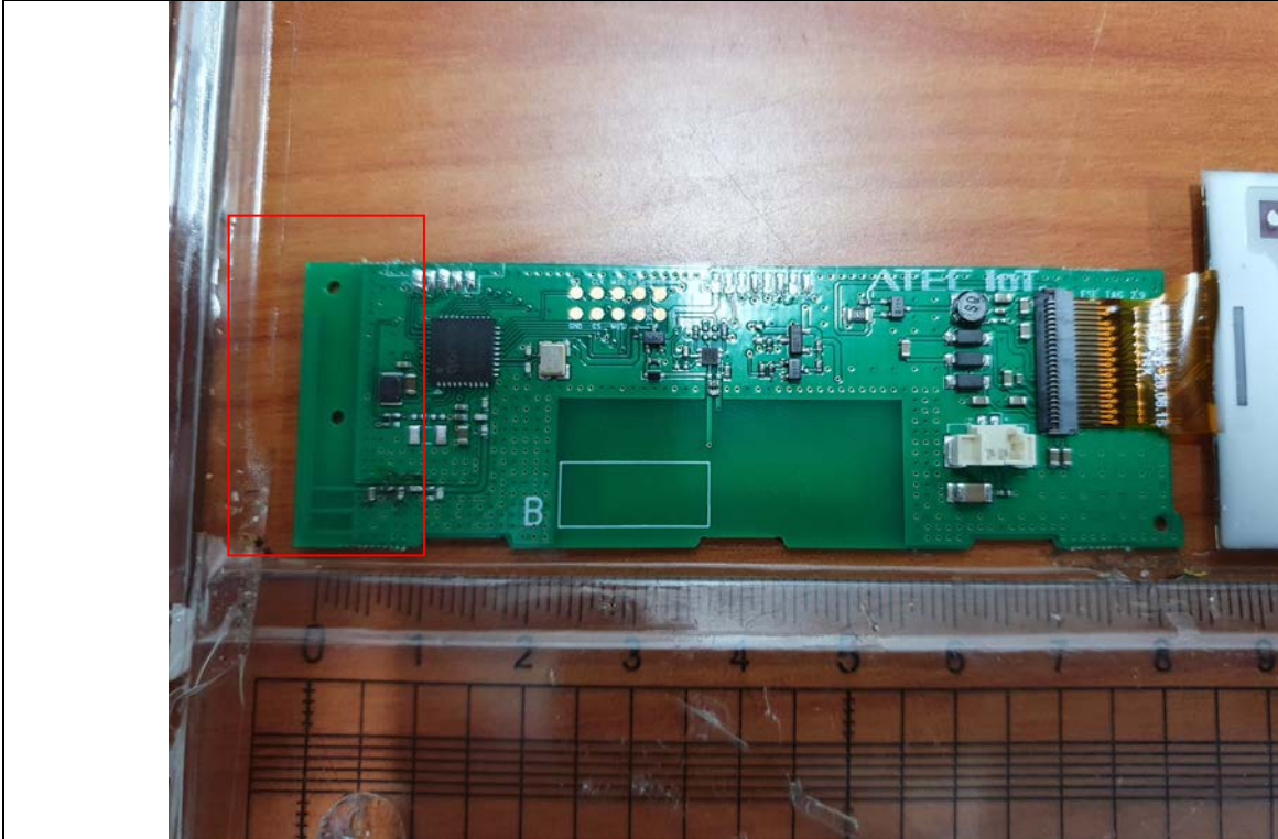
ANTENNA(2.4 GHz)
