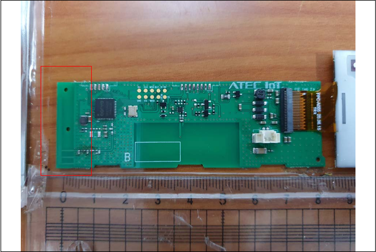
ANTENNA(2.4 GHz)
