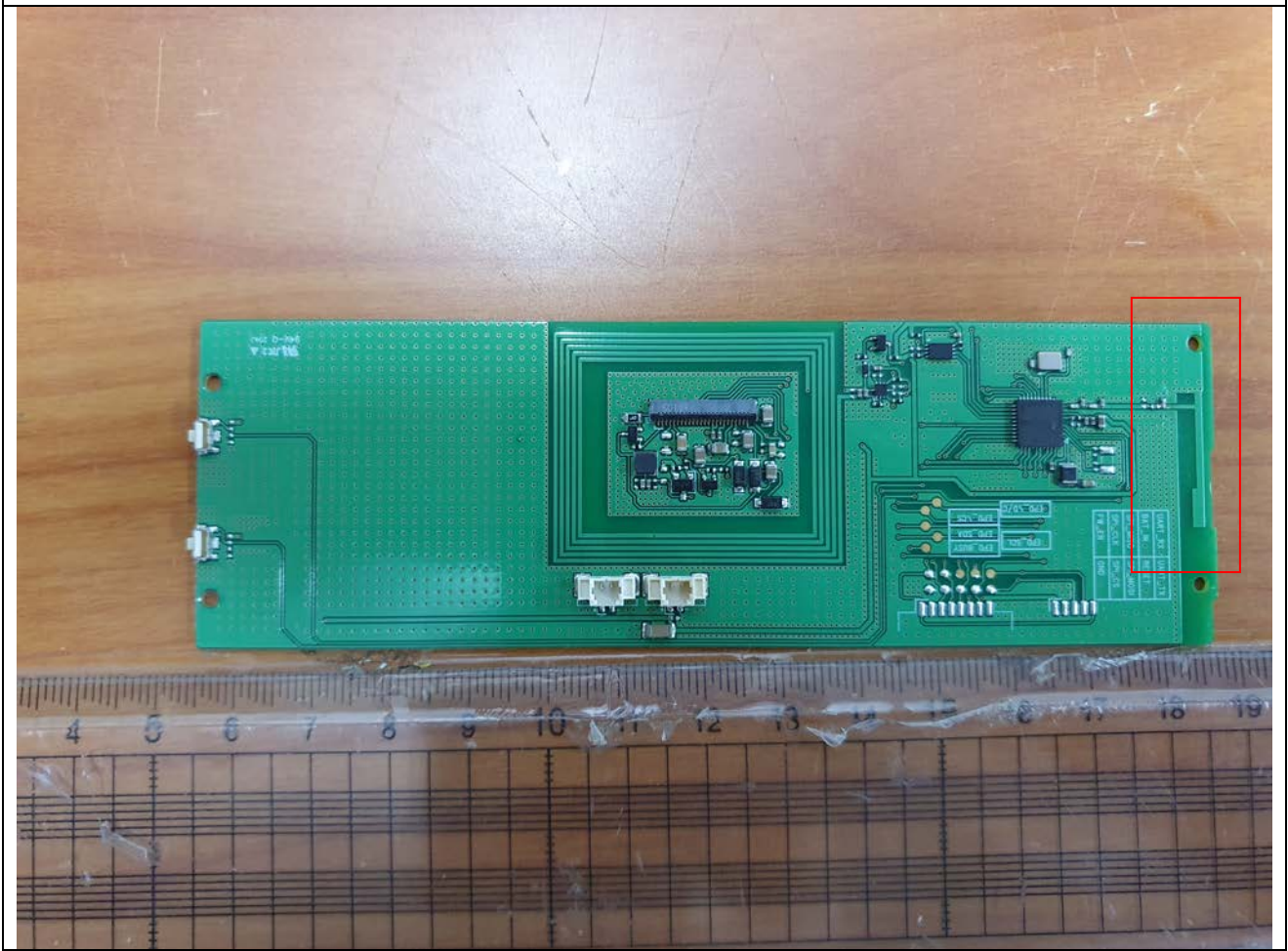
ANTENNA(2.4 GHz)
