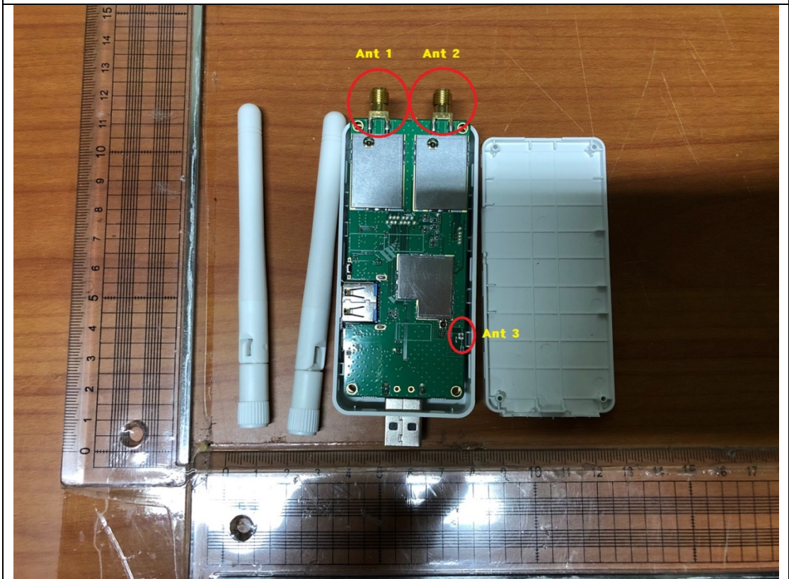
ANTENNA(2.4 GHz)
