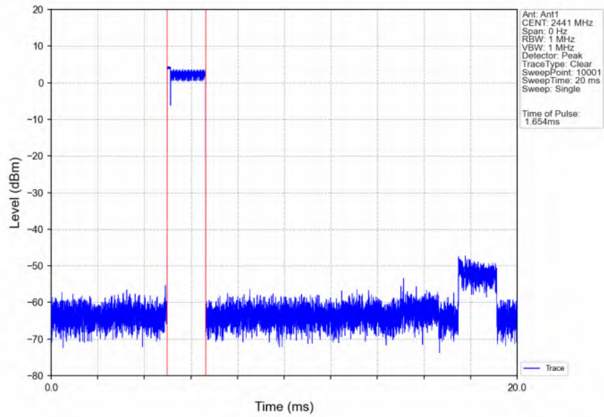
Pi/4DQPSK_2DH3_HOPP_Ant1_NTNV
